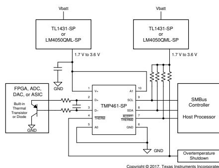
简化框图
