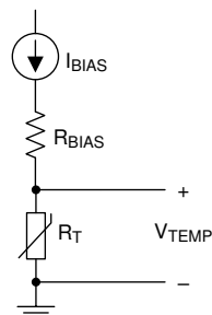
Figure 16. 线性热敏电阻的电流偏置电路
