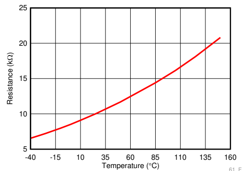
典型电阻与环境温度间的关系
