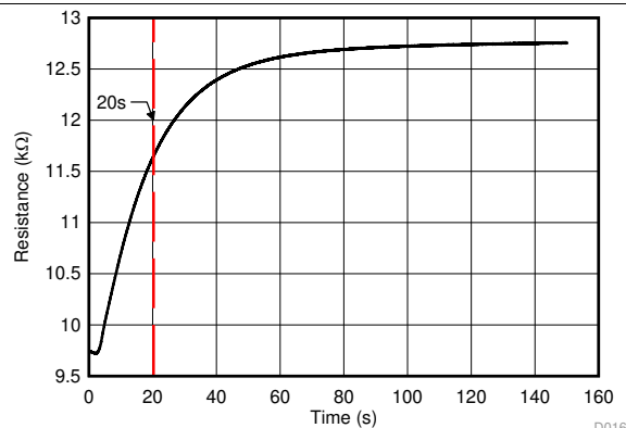
图 10. 热响应时间
