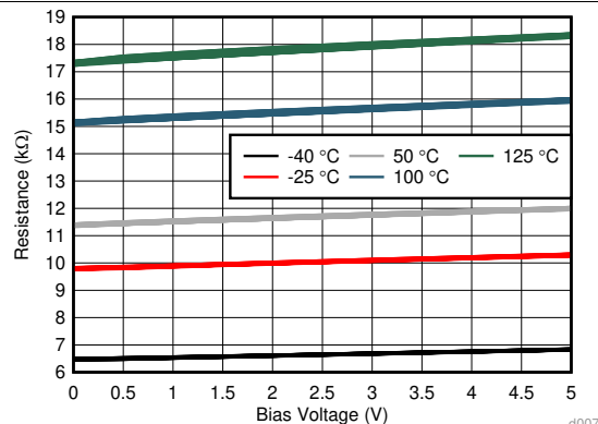
图 8. 电源相关电阻与偏置电压间的关系
