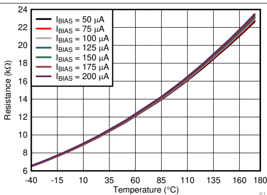
图 1. 多个偏置电流条件下电阻与环境温度间的关系
