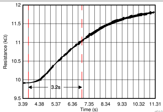
图 9. 阶跃响应
