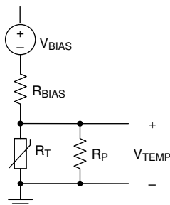
Figure 15. 线性热敏电阻的电压偏置电路
