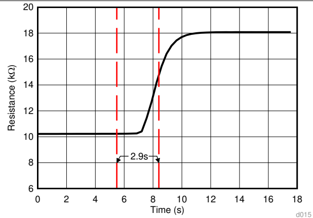
图 13. 热响应时间 ( LPG 封装 )
