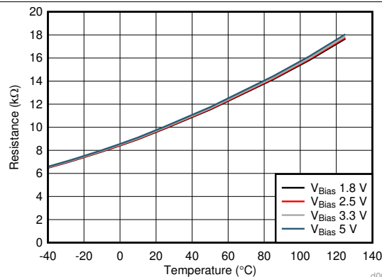
图 2. 多个偏置电压条件下电阻与环境温度间的关系
