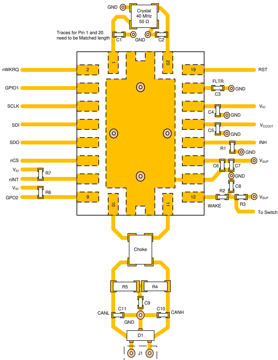
图 11-1. Example Layout
