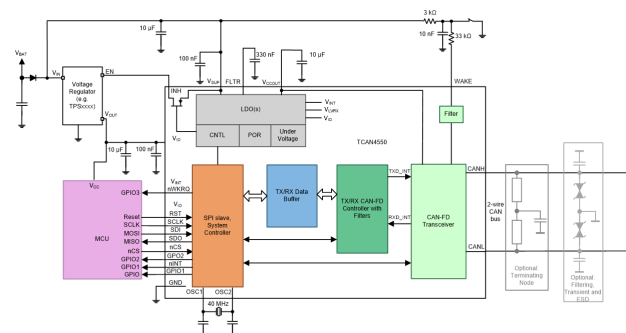
简化版原理图, 晶振
