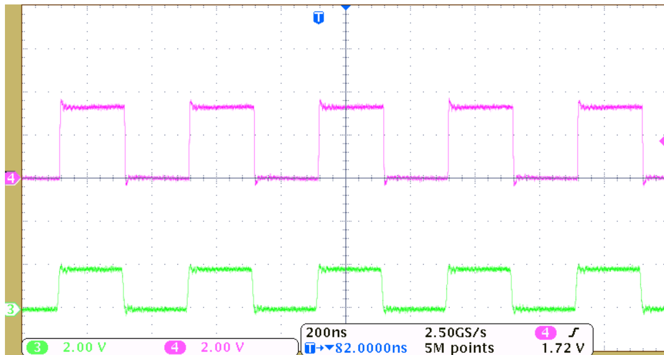
图 10. Level-Translation of a 2.5-MHz Signal
