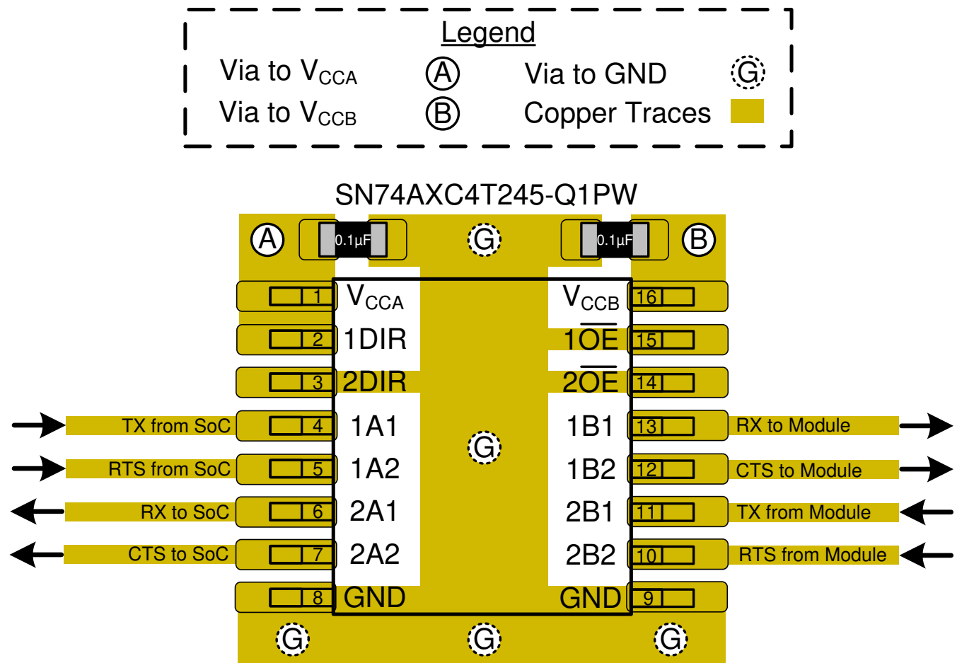
图 12. Layout Example
