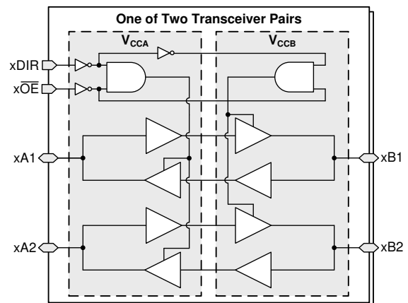
功能方框图
