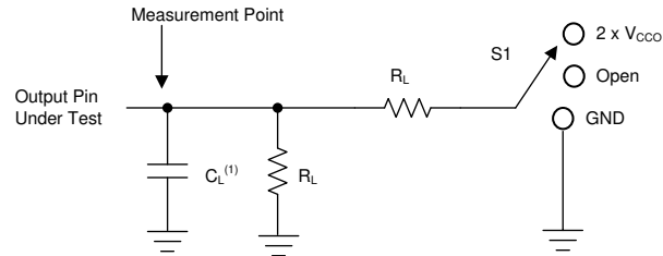
图 5. Load Circuit
