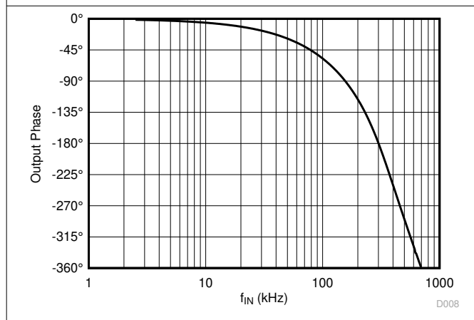
图 6-21. Output Phase vs Input Frequency
