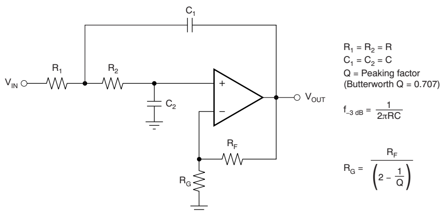
图 24. 两极低通 Sallen-Key 滤波器
