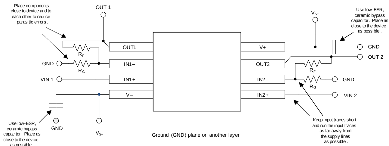
图 28. 布局示例
