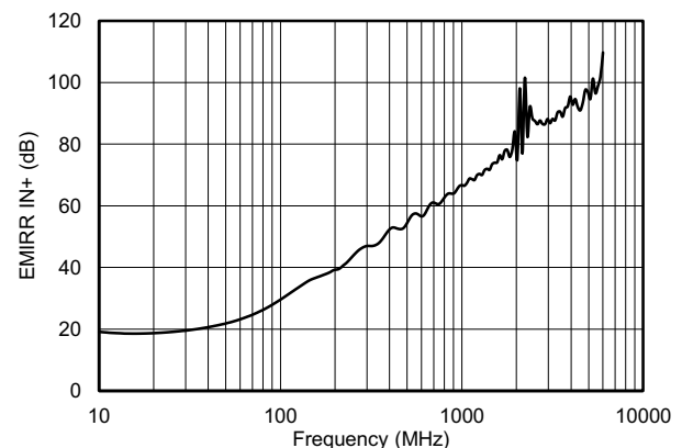
EMIRR IN+ 与频率间的关系
