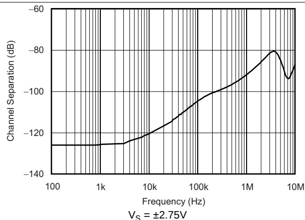
图 12. 通道分离与频率间的关系 (TLV2314)
