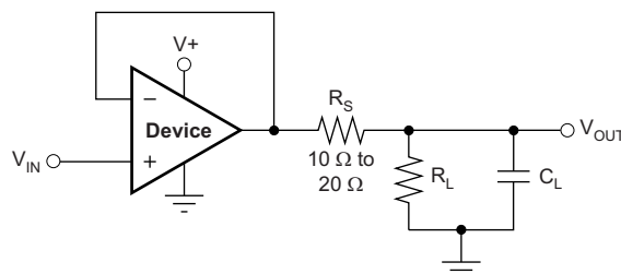
图 14. 改进容性负载驱动
