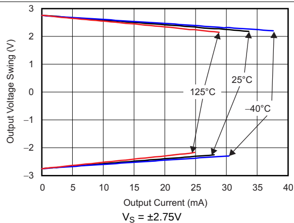
图 7. 输出电压摆幅与输出电流间的关系 (过热)
