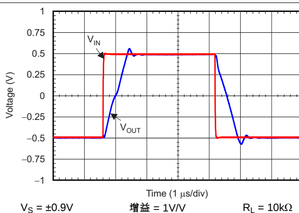
图 10. 大信号脉冲响应 (同相)
