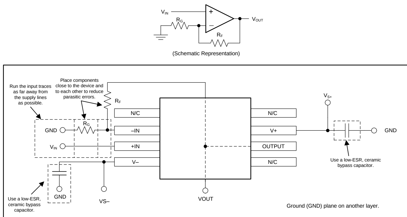
图 20. 同相配置的运算放大器电路板布局
