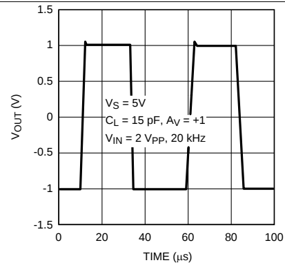
Figure 8. 大信号瞬态响应
