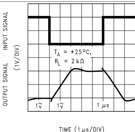
图 47. 反相大信号脉冲响应
