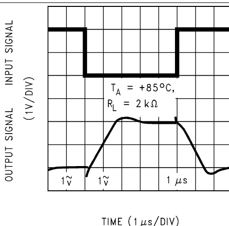
图 48. 反相大信号脉冲响应
