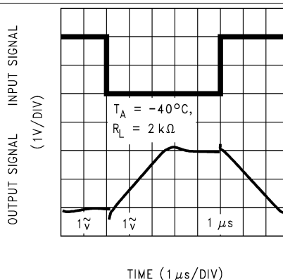
图 46. 反相大信号脉冲响应
