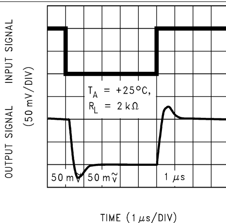
图 50. 同相小信号脉冲响应
