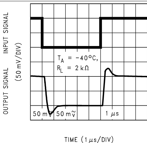
图 49. 同相小信号脉冲响应
