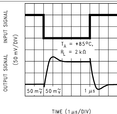
图 45. 反相小信号脉冲响应
