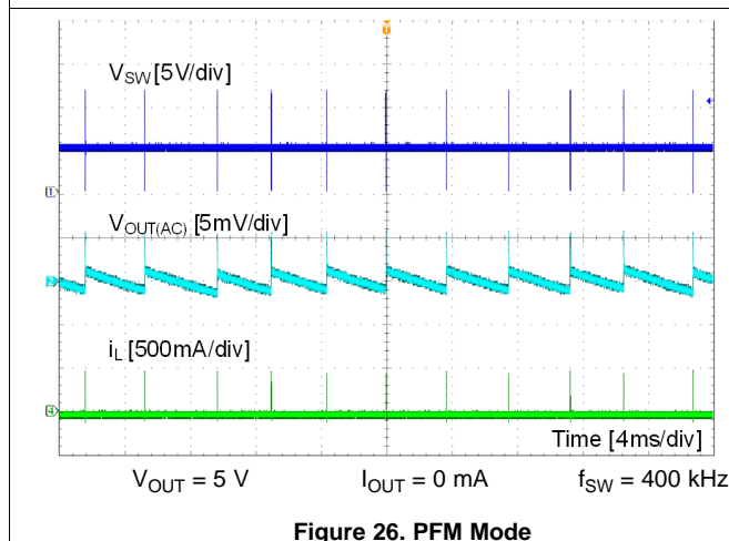
Figure 26. PFM Mode
