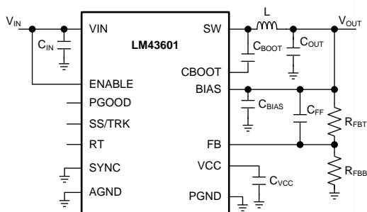
简化原理图
