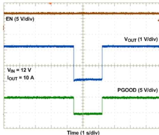
图 9-9. Overtemperature Protection
