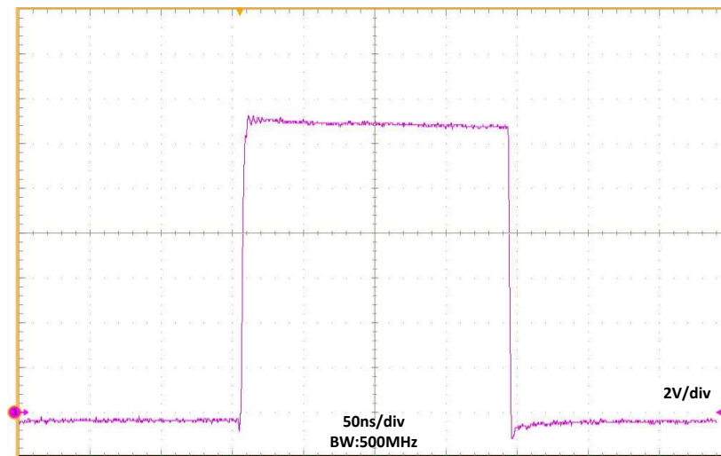
图 8. Switch Node Waveform
