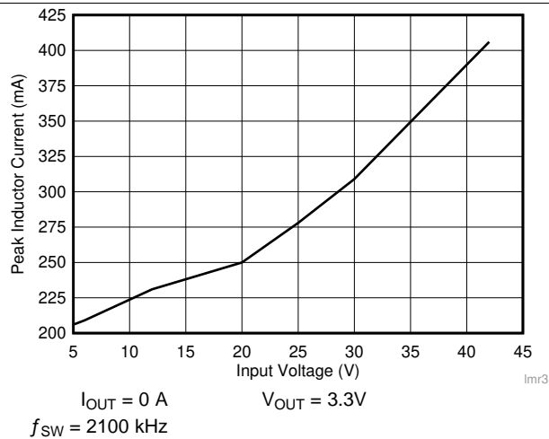
图 7. I PEAK-MIN
