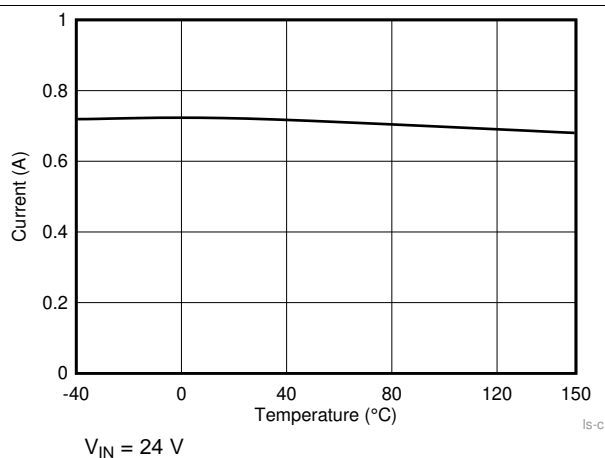
图 5. Low Side Current Limit
