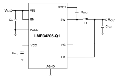
图 1. 简化原理图
