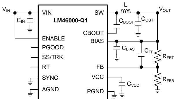
简化原理图
