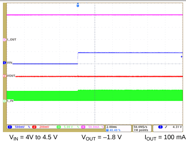
图 20. Line Step
