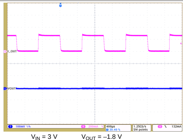
图 21. Load Step
