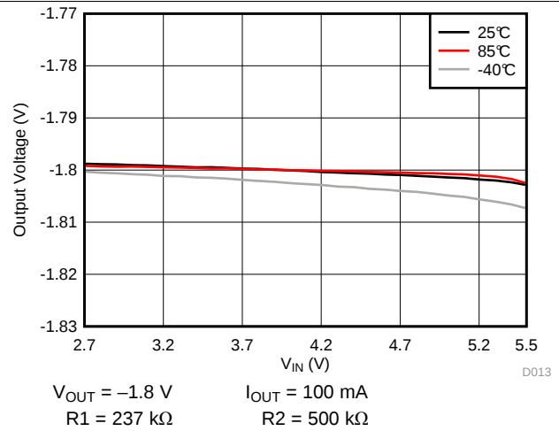
图 14. Line Regulation
