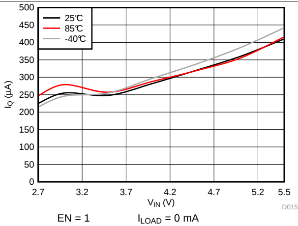
图 3. Quiescent Current
