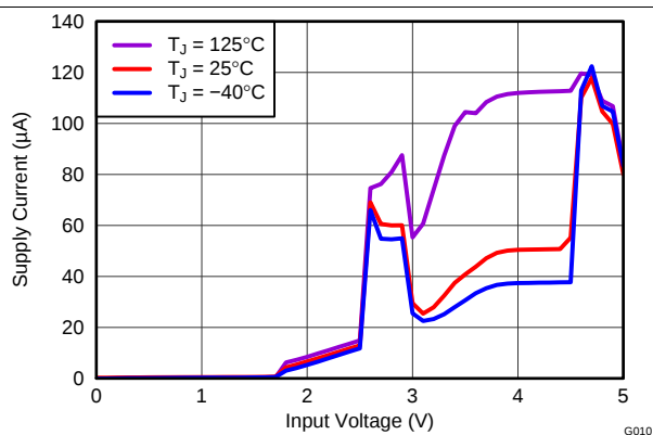
Figure 15. 电源电流 (VIN 引脚) 与输入电压 (0V 至 VSTART) 间的关系 (EN 引脚开路)
