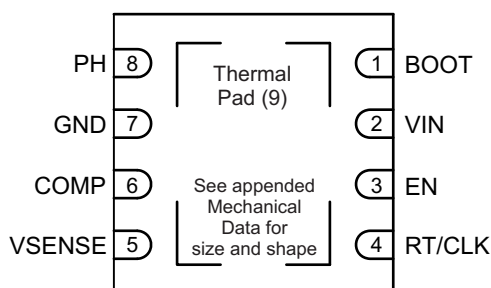
引脚功能
