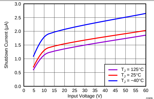
Figure 12. 关断电源电流 (I_VIN) 与输入电压间的关系
