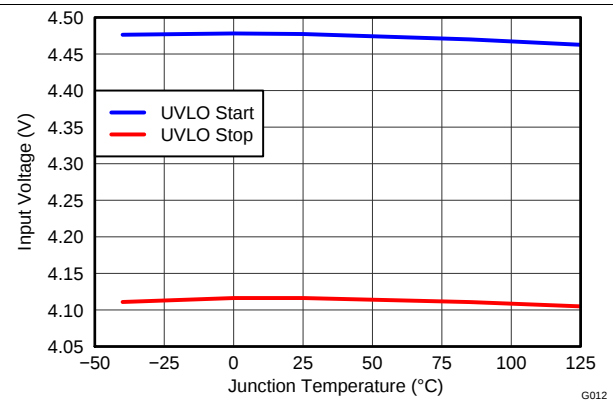
Figure 10. 输入电压 (UVLO) 与温度间的关系
