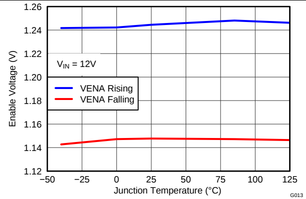
Figure 8. 使能引脚电压与温度间的关系
