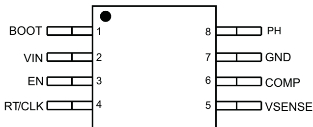
MSOP 封装 8 引脚 俯视图
