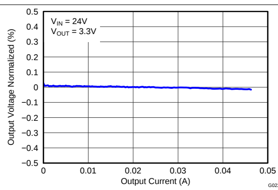
Figure 40. 输出电压与输出电流间的关系
