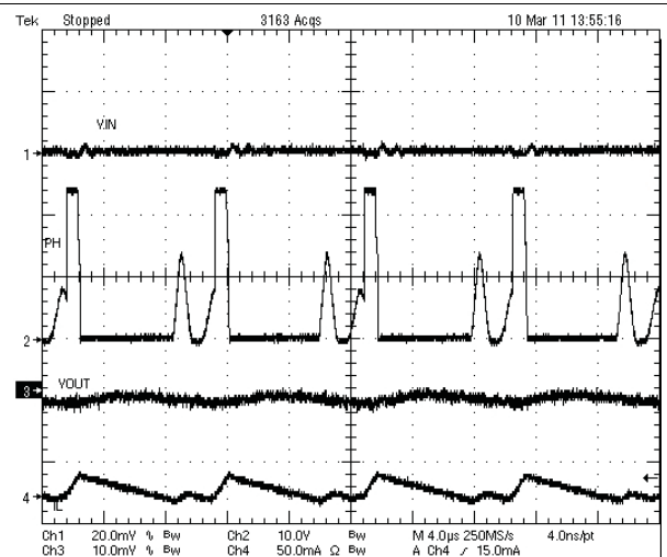
Figure 48. DCM 下的输入和输出纹波
