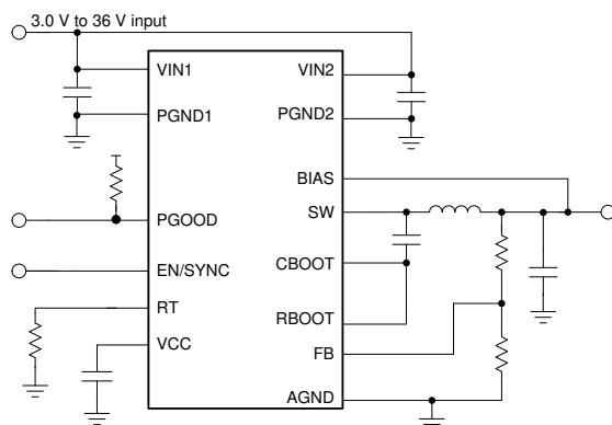
简化原理图
