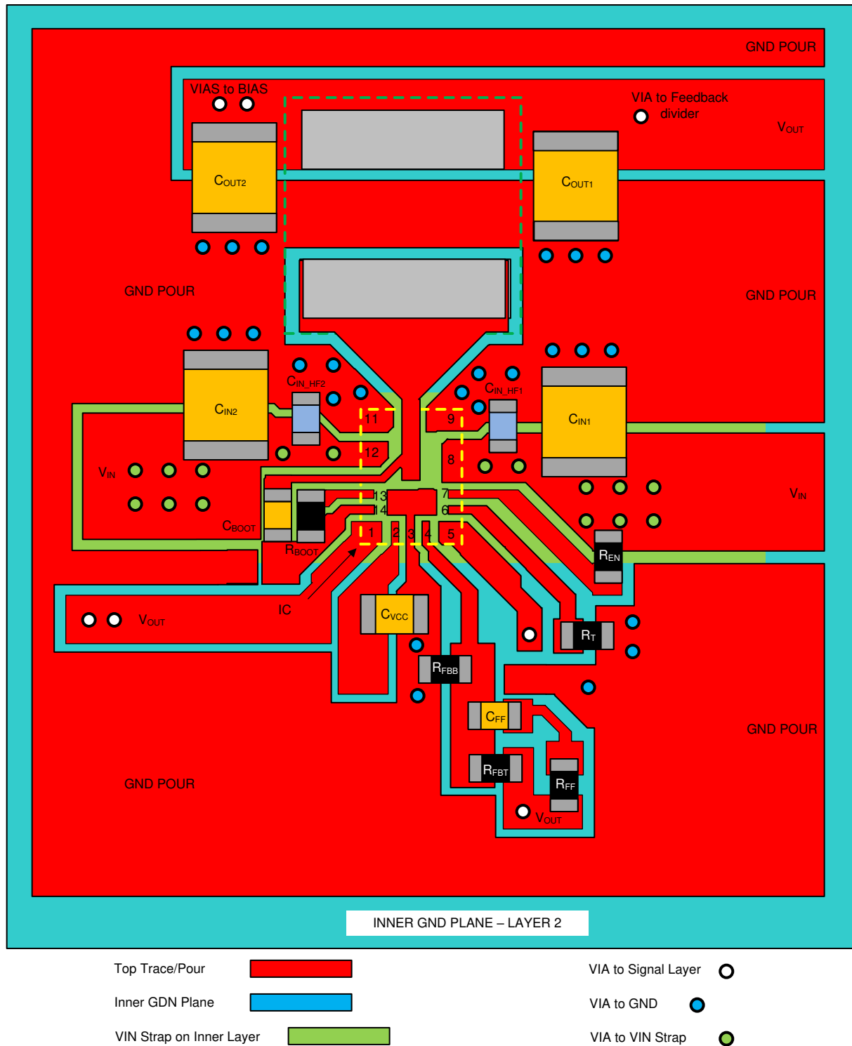
图 78. Layout Example
