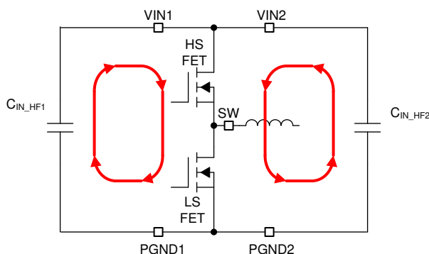
图 77. Input Current Loop
