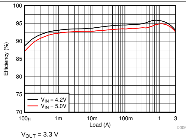
图 15. Efficiency
