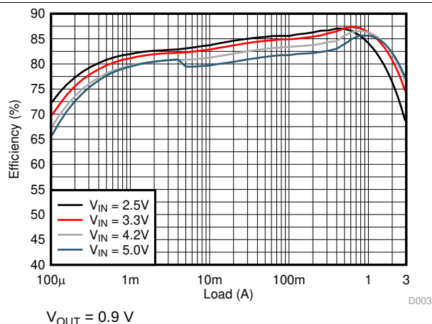
图 9. Efficiency
