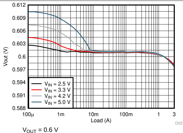
图 8. Load Regulation
