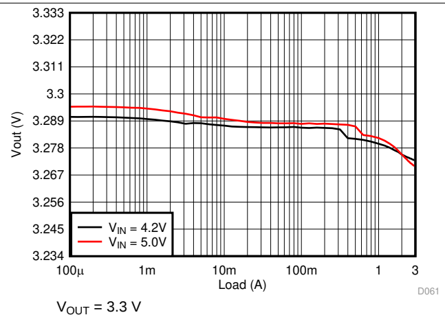
图 16. Load Regulation
