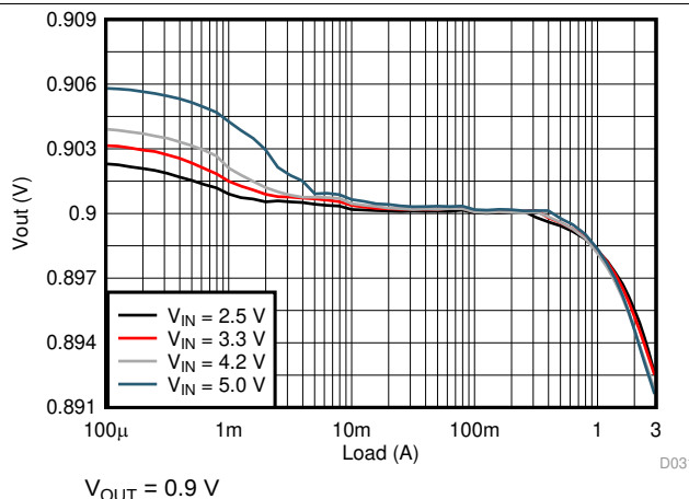
图 10. Load Regulation
