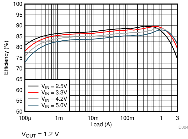
图 11. Efficiency
