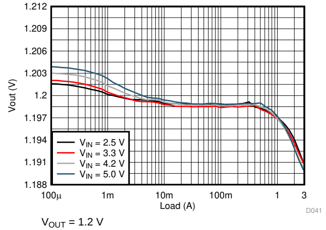
图 12. Load Regulation
