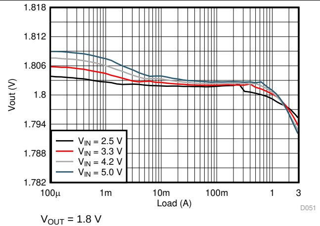
图 14. Load Regulation
