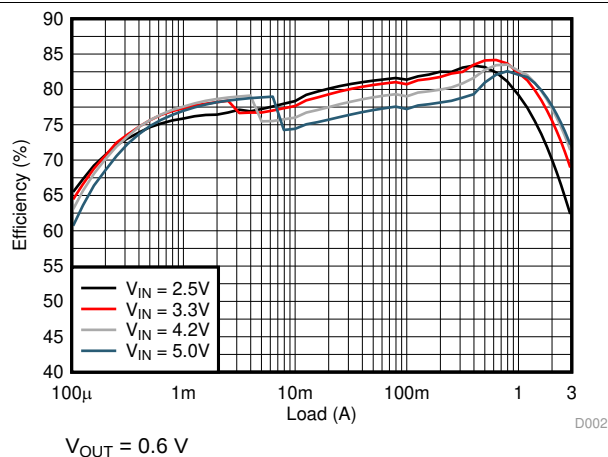
图 7. Efficiency
