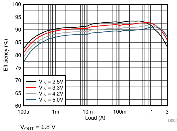
图 13. Efficiency
