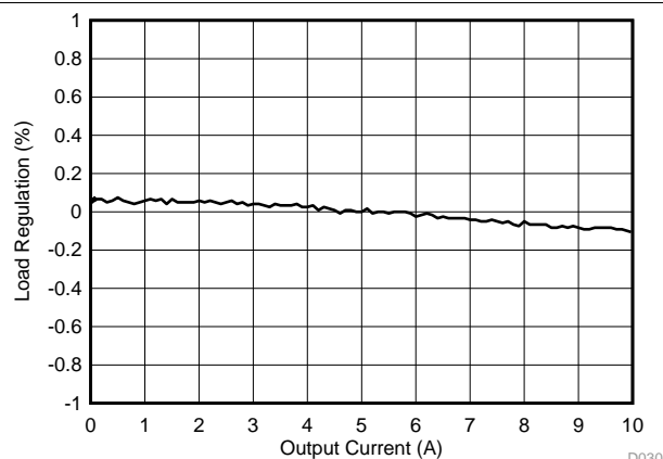
图 50. Load Regulation
