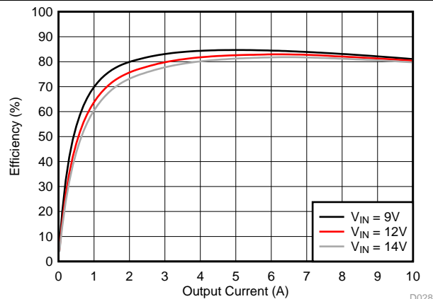
图 48. Efficiency
