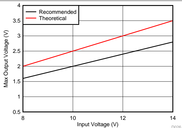
图 24. Max Output Voltage vs Input Voltage
