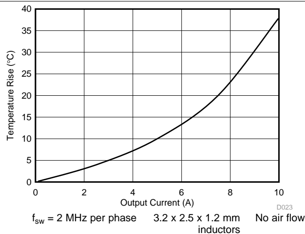
图 21. Case Temperature Rise vs Output Current
