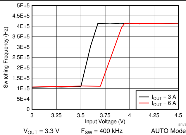
图 55. LM61460-Q1 Frequency Dropout
