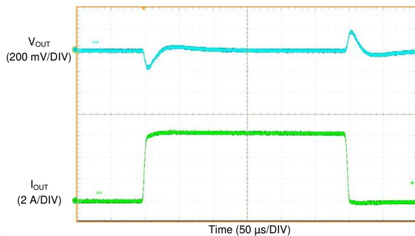
图 73. LM61460-Q1 Load Transient
