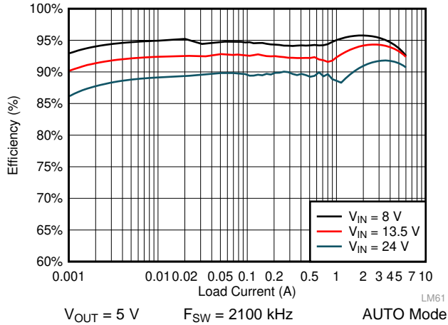
图 41. LM61460-Q1 Efficiency
