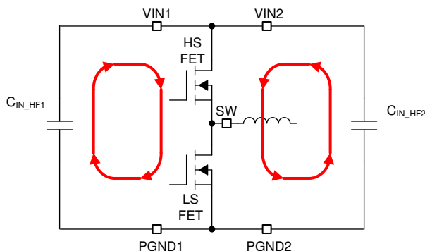
图 87. Input Current Loop
