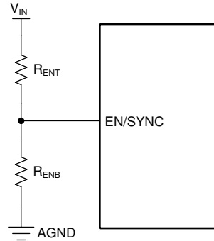
图 34. UVLO Using EN
