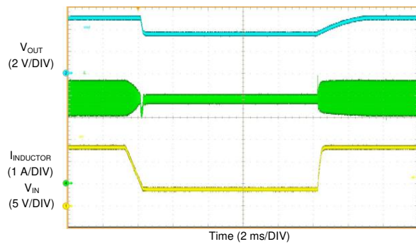
图 65. LM61460-Q1 Short Circuit Recovery
