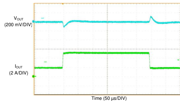
图 68. LM61460-Q1 Load Transient
