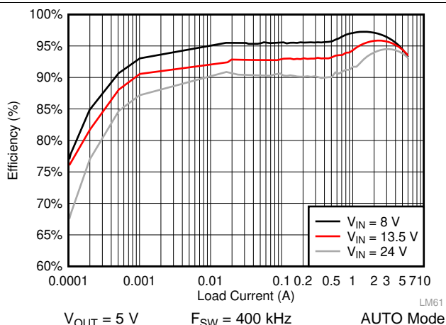
图 39. LM61460-Q1 Efficiency
