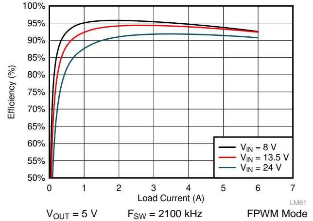
图 42. LM61460-Q1 Efficiency
