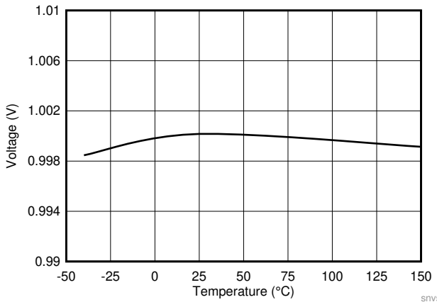
图 3. Feedback Voltage
