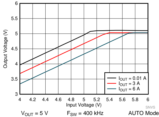
图 53. LM61460-Q1 Dropout Curve
