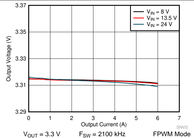
图 46. LM61460-Q1 Load and Line Regulation
