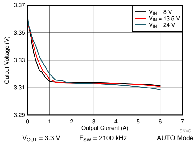
图 45. LM61460-Q1 Load and Line Regulation
