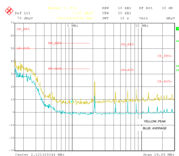
传导 EMI: V_{OUT} = 5V , I_{OUT} = 5A
