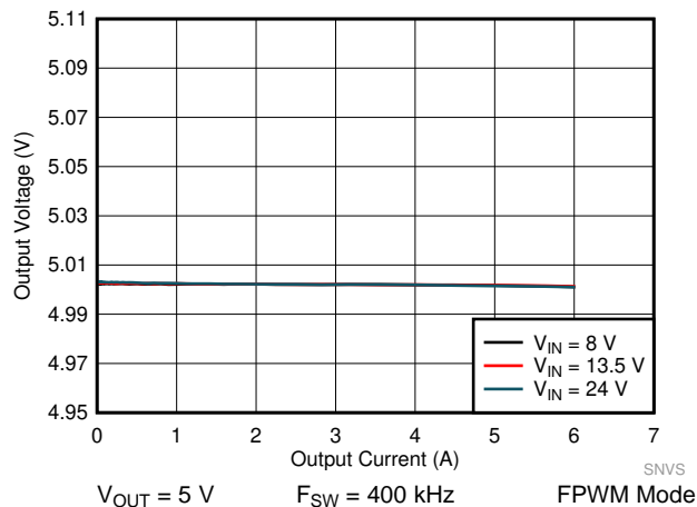
图 48. LM61460-Q1 Load and Line Regulation
