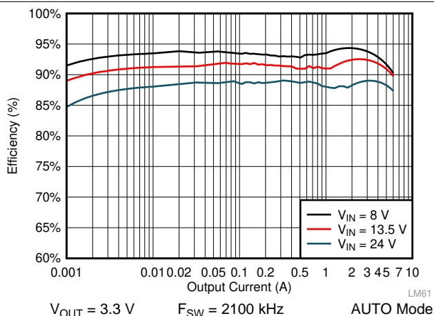
图 37. LM61460-Q1 Efficiency
