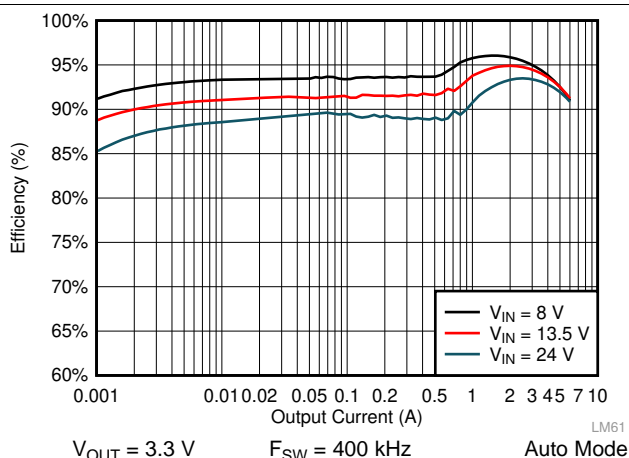
图 35. LM61460-Q1 Efficiency
