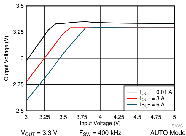
图 51. LM61460-Q1 Dropout Curve
