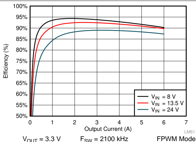
图 38. LM61460-Q1 Efficiency
