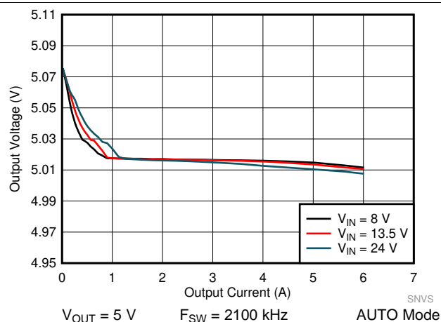
图 49. LM61460-Q1 Load and Line Regulation
