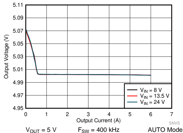
图 47. LM61460-Q1 Load and Line Regulation
