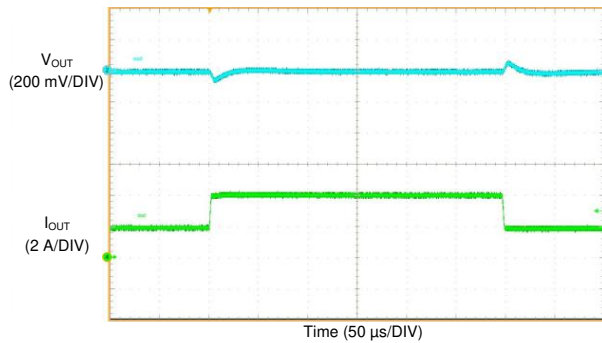
图 71. LM61460-Q1 Load Transient
