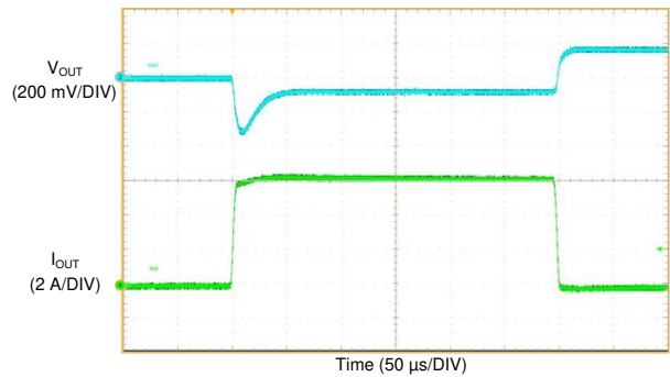
图 72. LM61460-Q1 Load Transient
