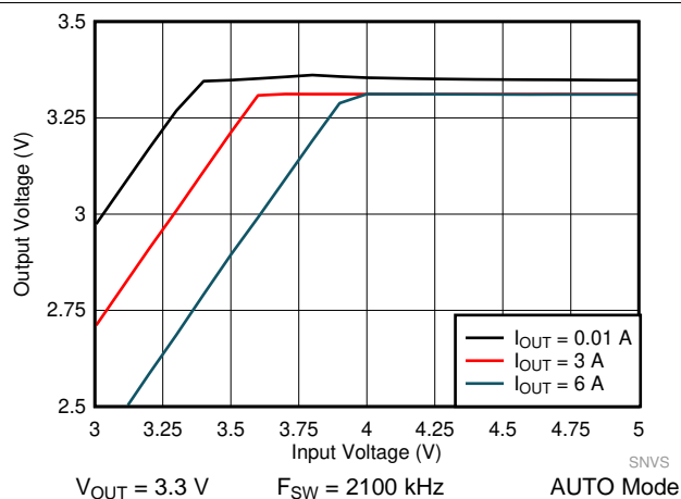
图 52. LM61460-Q1 Dropout Curve
