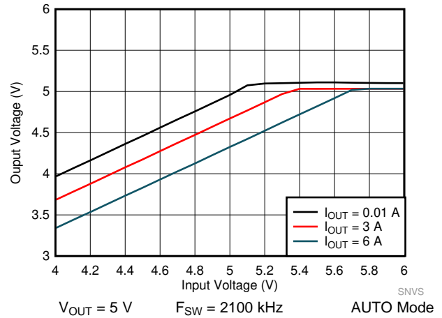
图 54. LM61460-Q1 Dropout Curve
