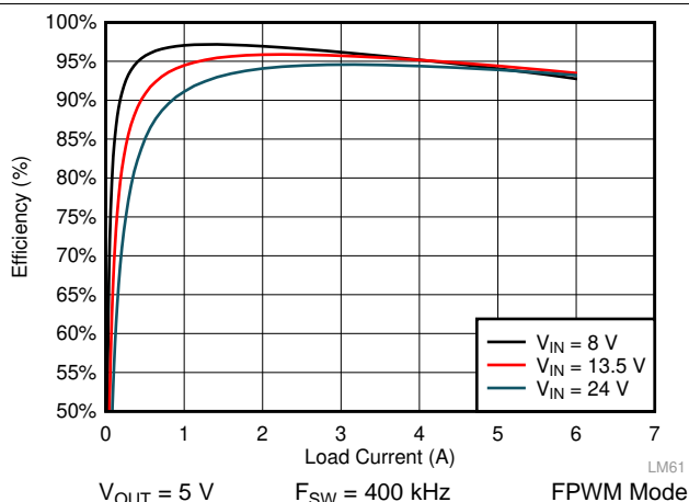
图 40. LM61460-Q1 Efficiency
