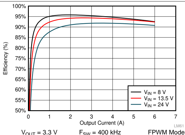
图 36. LM61460-Q1 Efficiency
