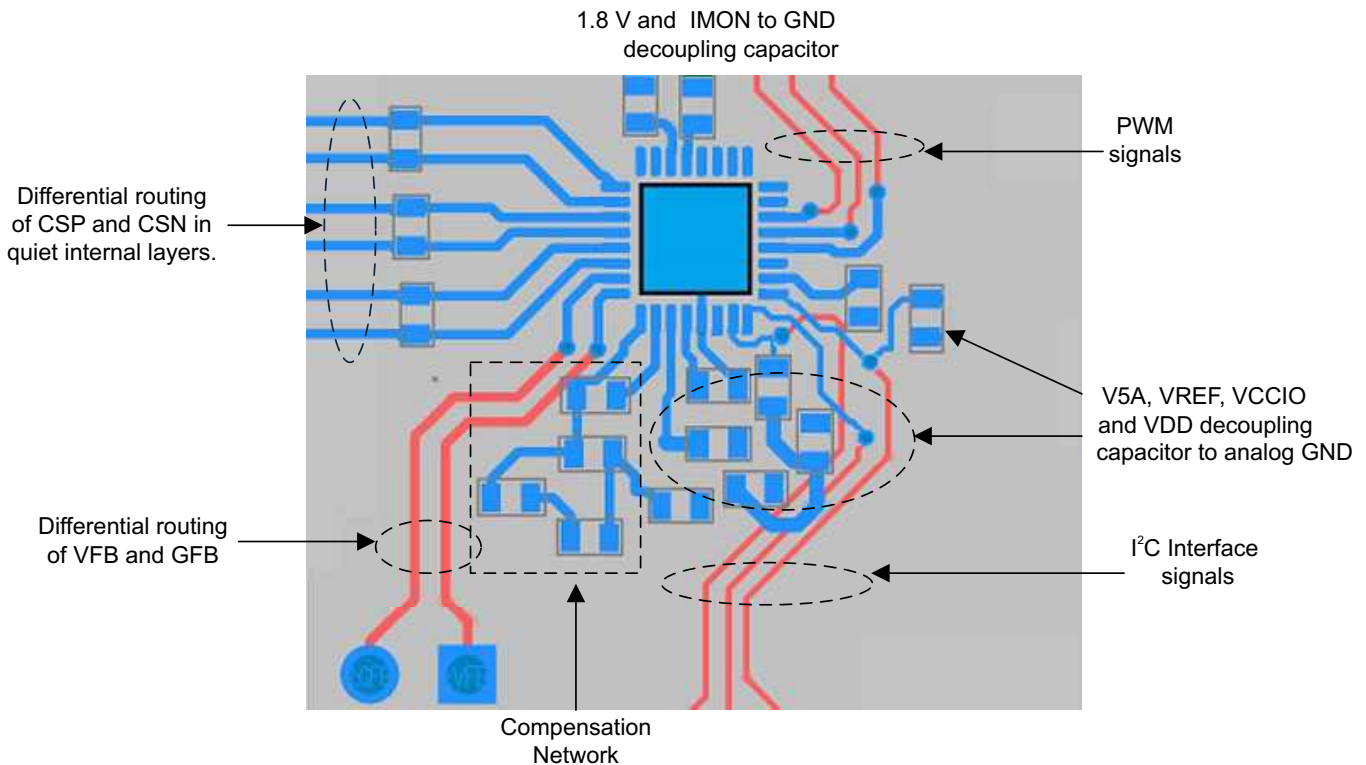
图 31. Example Layout
