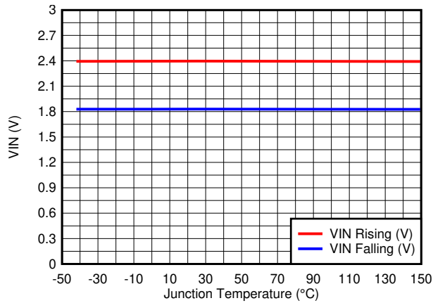
图 6-7. VIN UVLO
