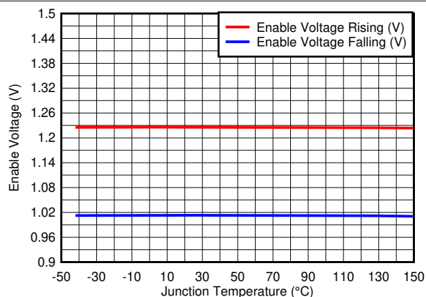
图 6-5. Enable Voltage
