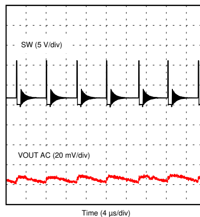
图 8-25. Output Voltage Ripple - DCM
