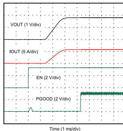
图 8-15. EN Start-Up
