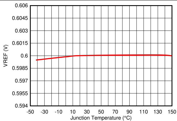
图 6-6. Vref
