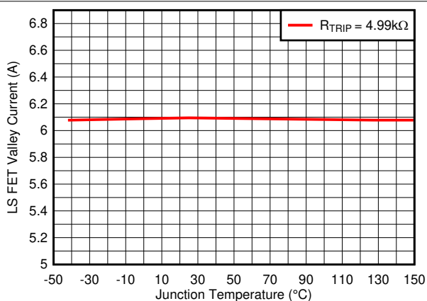
图 6-3. Overcurrent Limit
