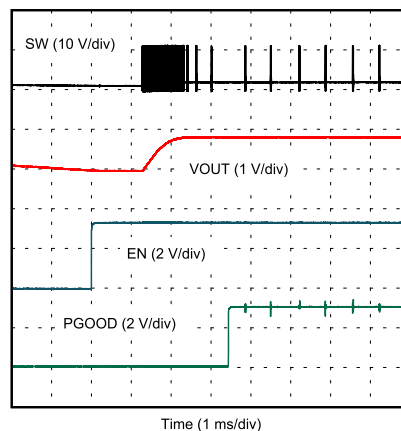
图 8-27. EN Start-Up With Prebias
