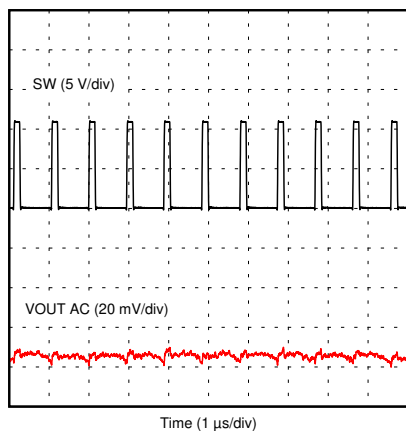
图 8-26. Output Voltage Ripple
