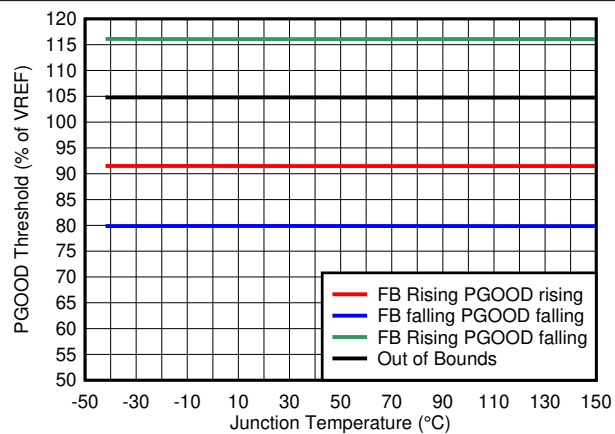
图 6-9. PGOOD Thresholds
