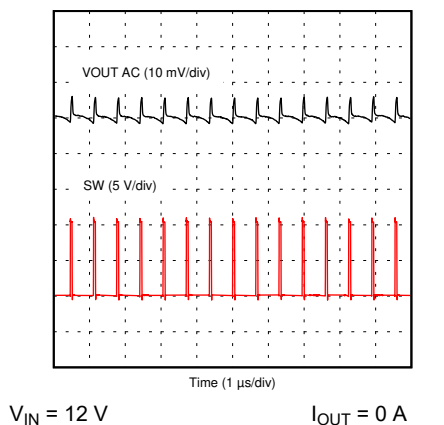
图 8-28. Output Ripple – No Load
