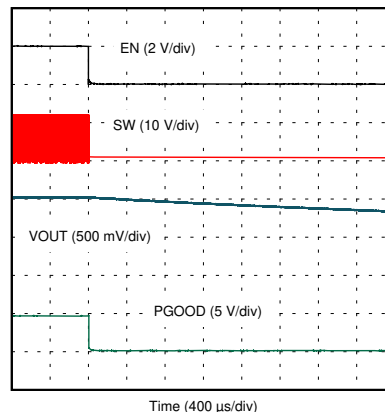
V_{IN} = 12\text{ V} I_{OUT} = 0\text{ A} 图 8-11. EN Shutdown
