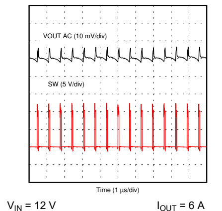
图 8-29. Output Ripple – 6-A Load
