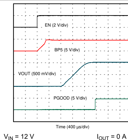
图 8-9. EN Start-up - Measuring BP5
