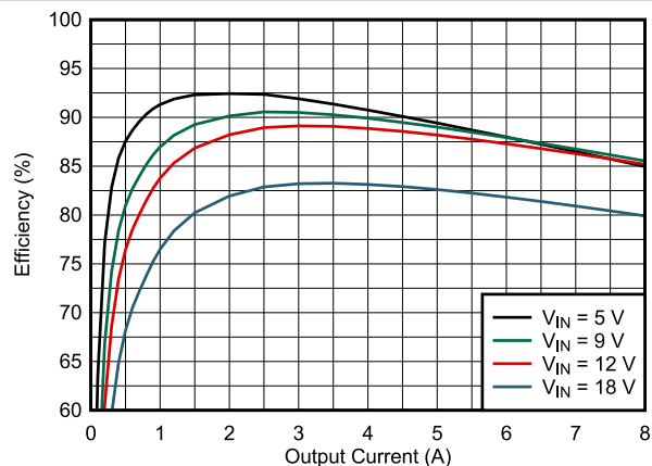
图 8-4. Efficiency
