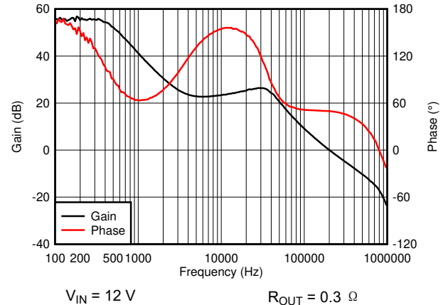
图 8-27. Bode Plot
