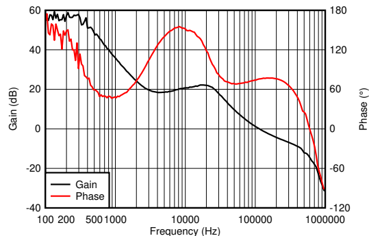
图 8-34. Bode Plot
