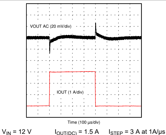
图 8-8. Load Transient
