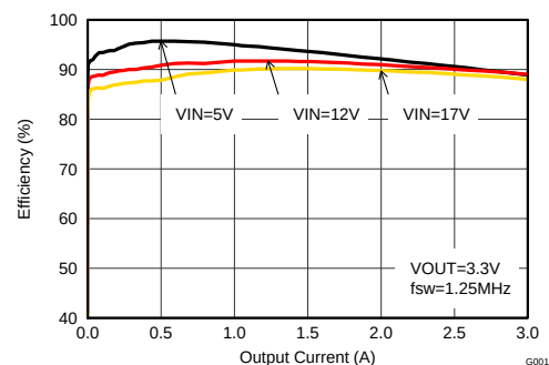
效率与输出电流
