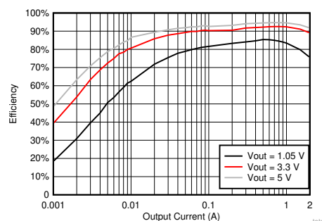
TPS562202S 效率
