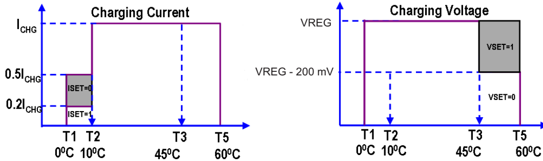
图 15. Charging Values
