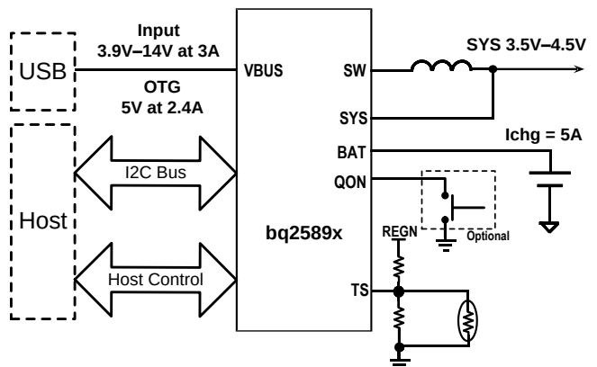
简化原理图
