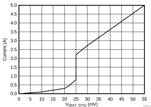
图 12. BATFET V-I Curve
