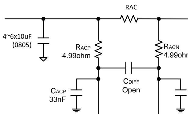
图 47. ACN-ACP Input Filter
