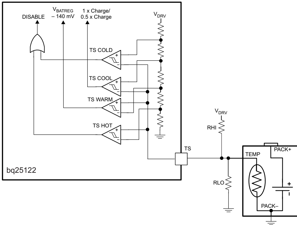
图 18. TS Circuit
