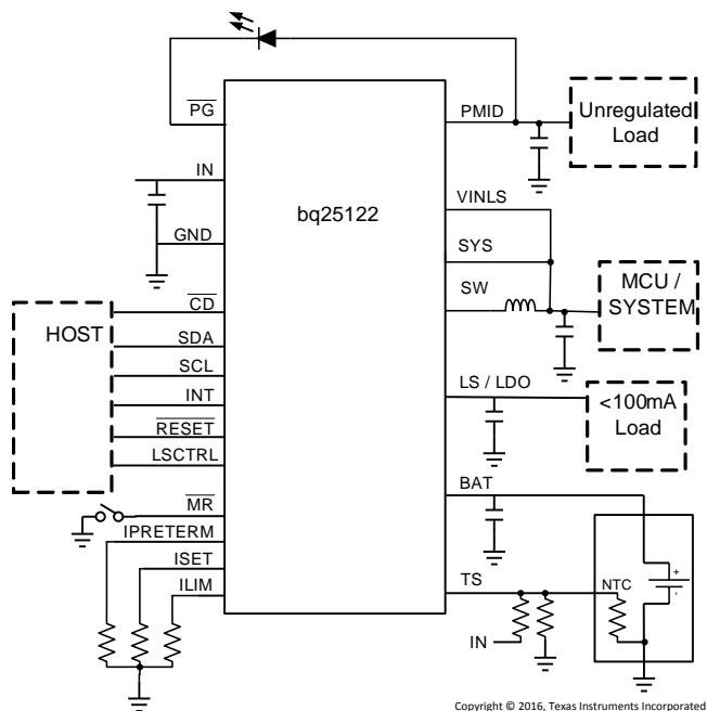
简化电路原理图
