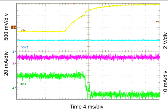
图 45. OVP Fault
