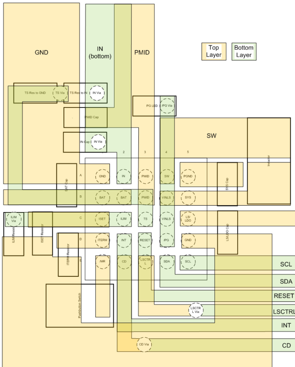
图 105. bq25122 Layout
