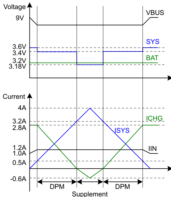
图 12. DPM Response
