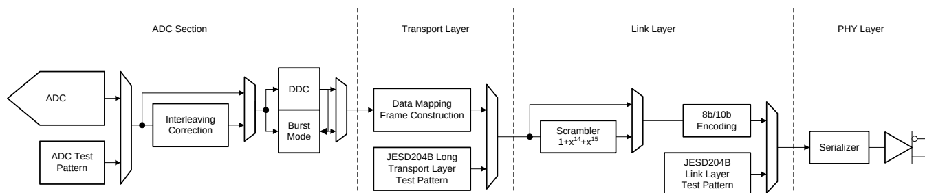
图 134. ADC Test Pattern
