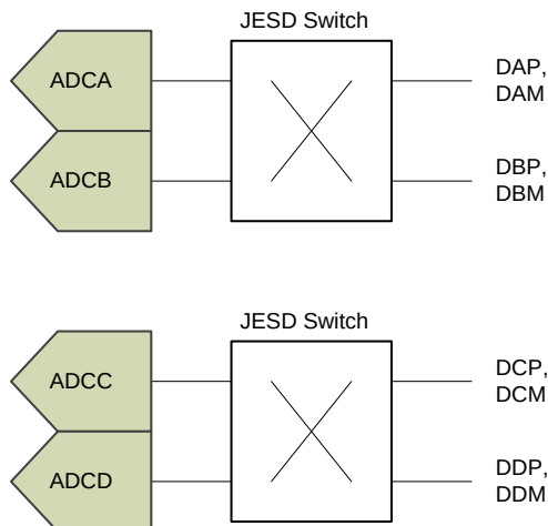
图 66. Switching the Output Lanes
