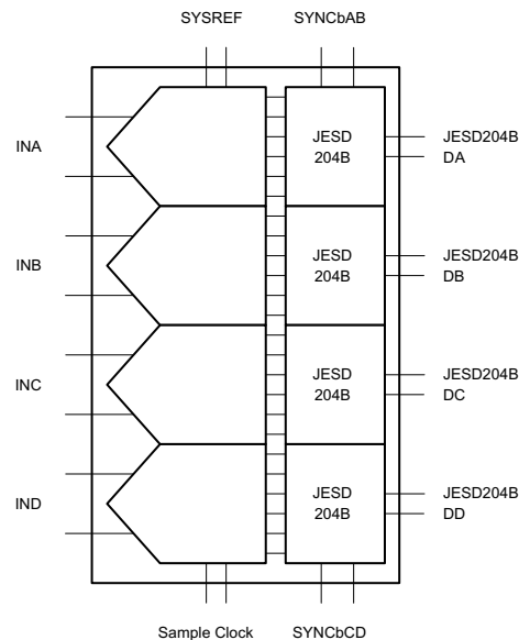
图 63. JESD204B Transmitter Block
