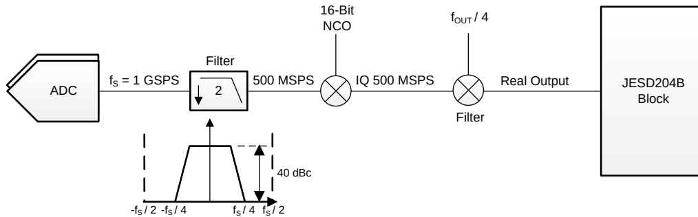
图 54. Operating Mode 3
