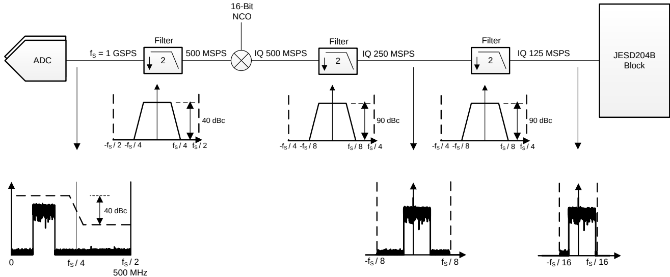
图 56. Operating Mode 6
