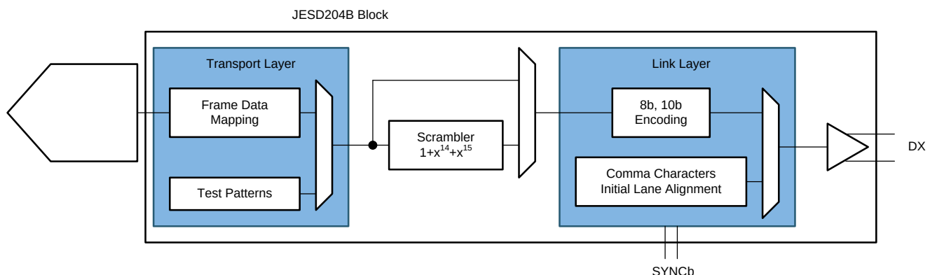
图 64. JESD Interface Block Diagram
