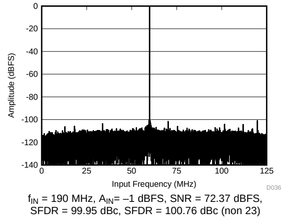
图 37. FFT for 190-MHz Input Signal
