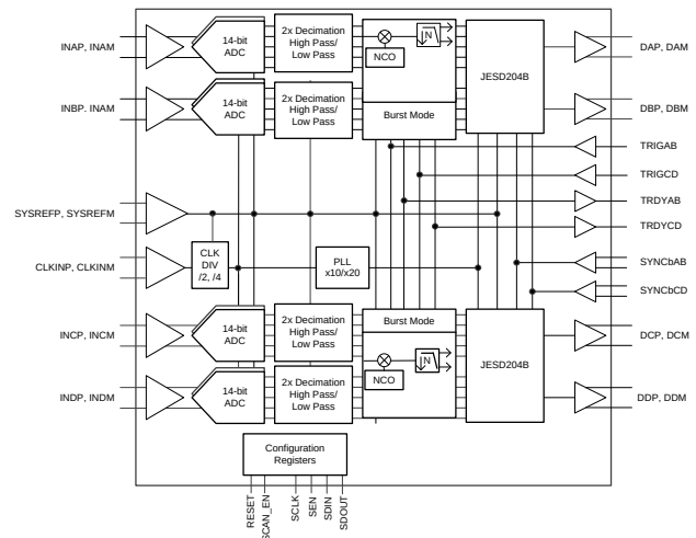
简化框图
