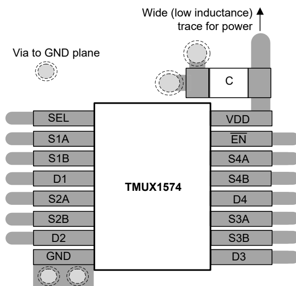
图 46. Example Layout
