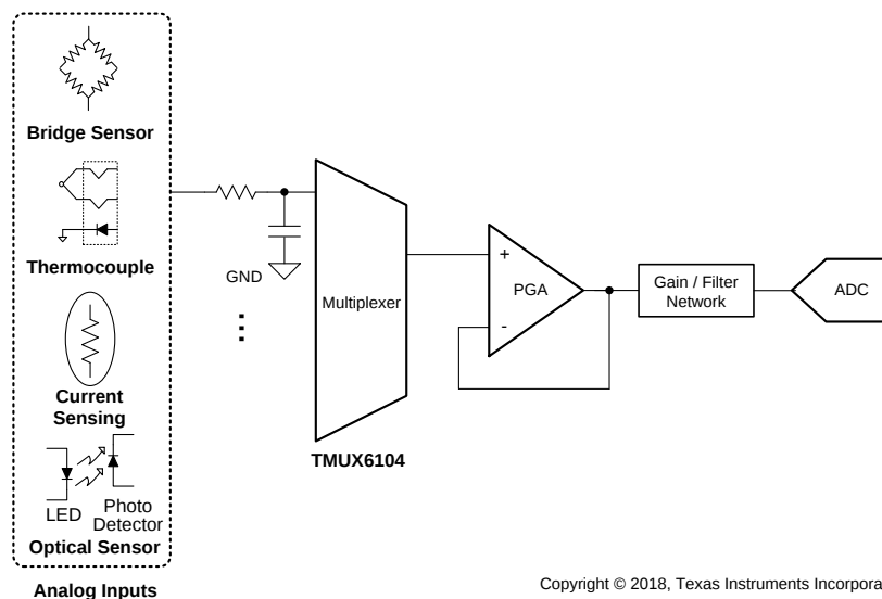
简化原理图
