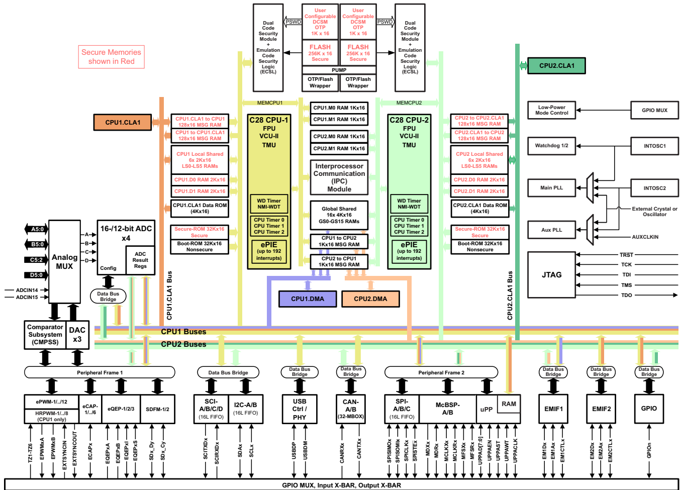
图 1-1. 功能方框图
