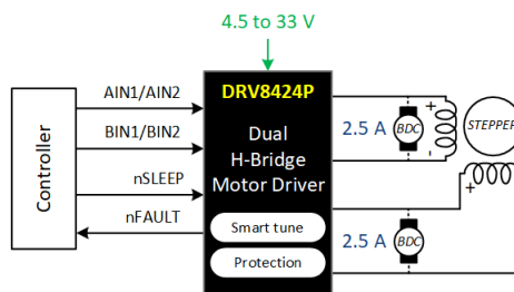
DRV8424P 简化原理图
