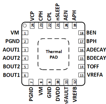
图 5-2. RGE 封装 24 引脚 VQFN ( 带有外露散热焊盘 ) 俯视图 ( DRV8424E 和 DRV8425E )
