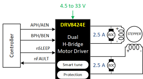
DRV8424E 简化原理图
