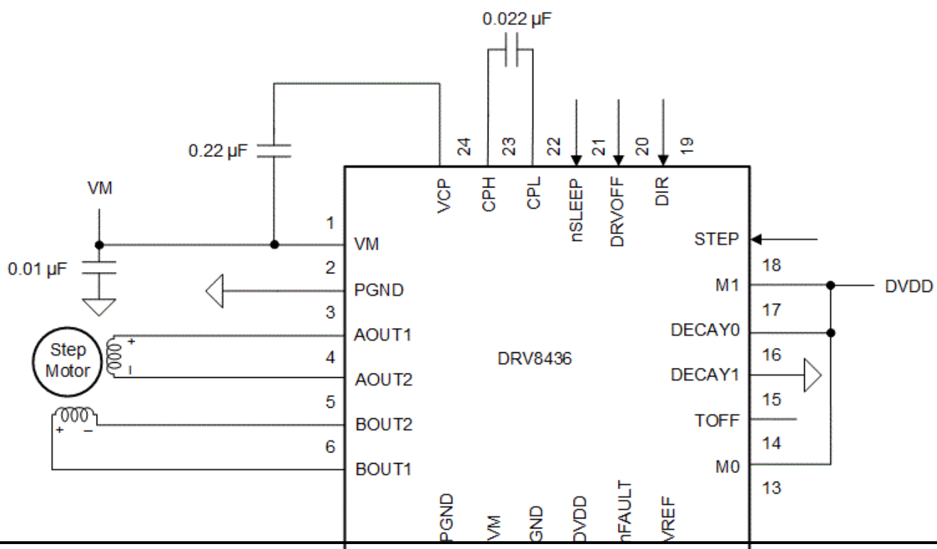
图 8-1. 典型应用原理图 ( HTSSOP 封装 )
