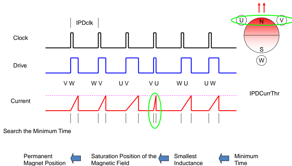
图 15. IPD Function
