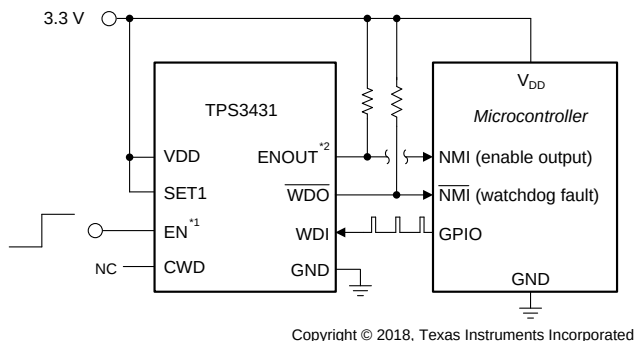
标准监视器计时器电路
