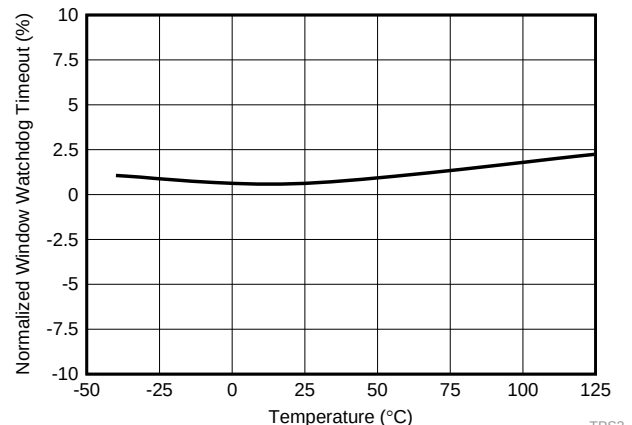
标准化监视器超时 ( t_{\text{WD}} ) 精度 (SET1 = 1, CWD = NC)
