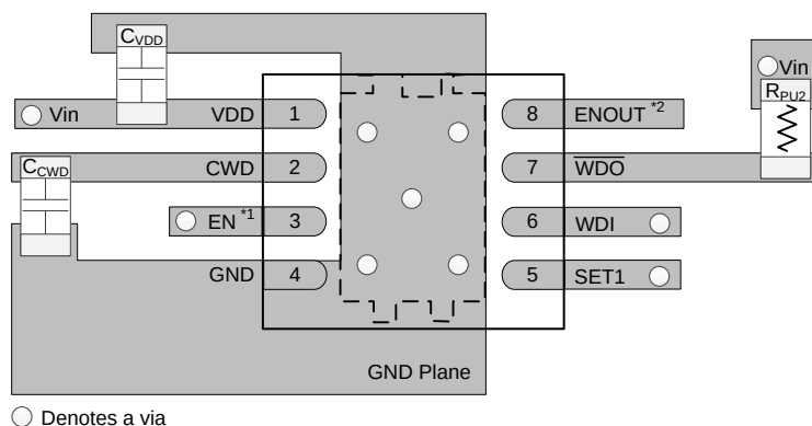
图 19. TPS3431-Q1 Recommended Layout
