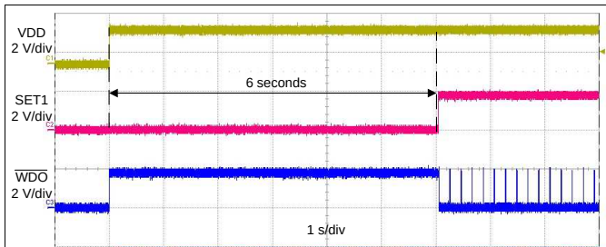
图 16. Startup Without a WDI Signal
