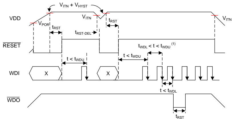
图 1. Timing Diagram
