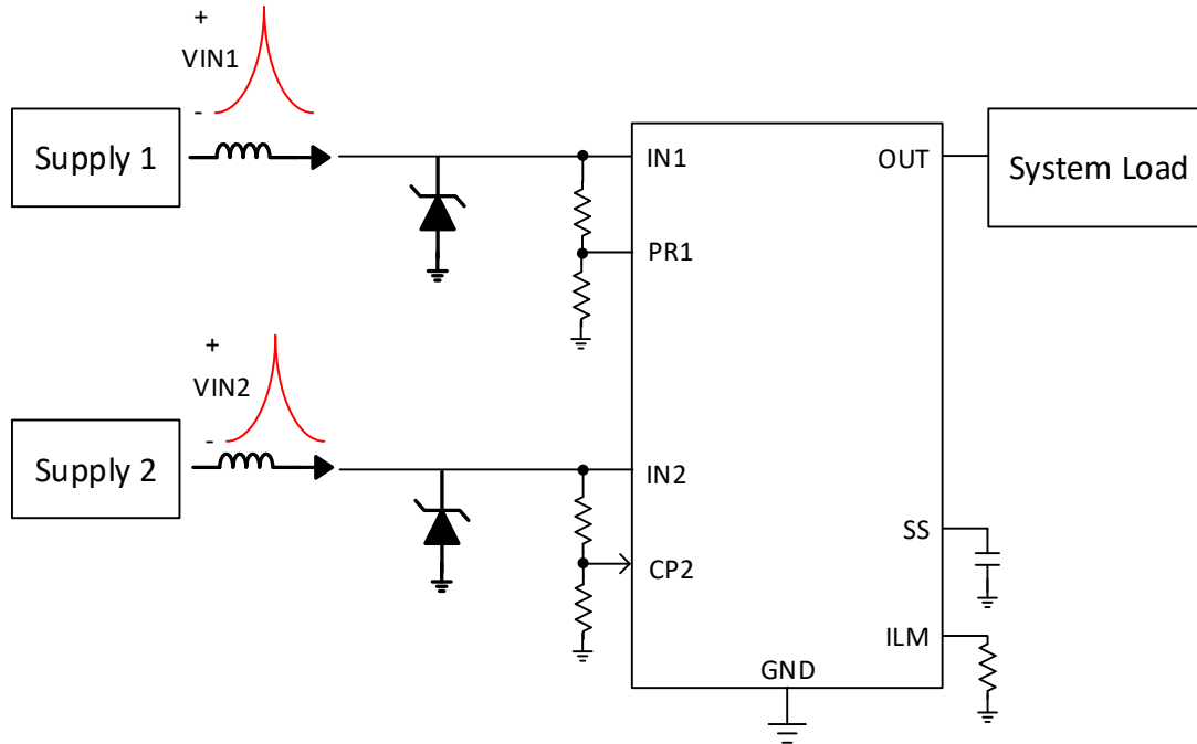
图 39. TPS212x Hotplug Configuration
