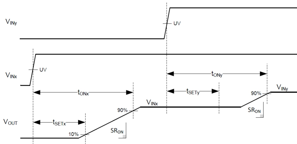
图 9. Timing Parameter Diagram
