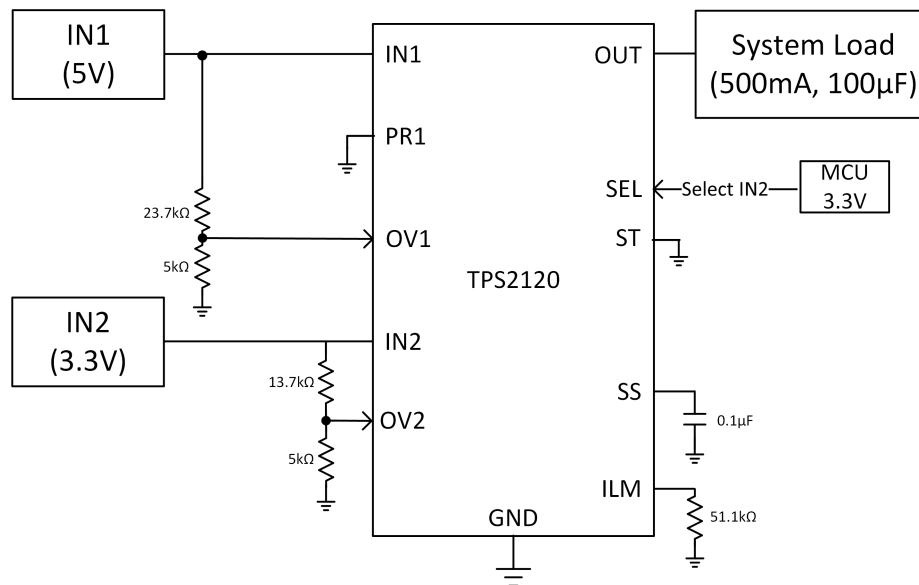
图 22. TPS2120 Manual Switchover
