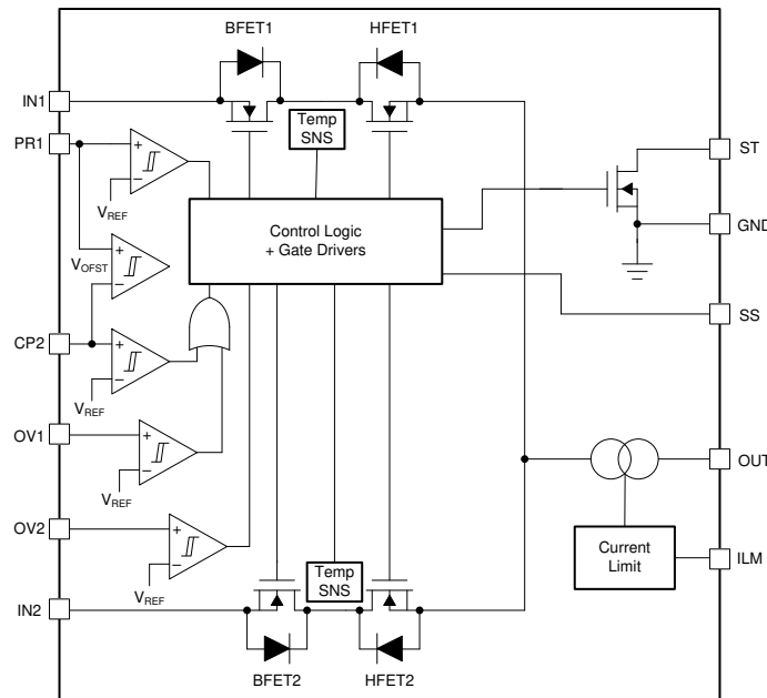
图 11. TPS2121 Functional Block Diagram
