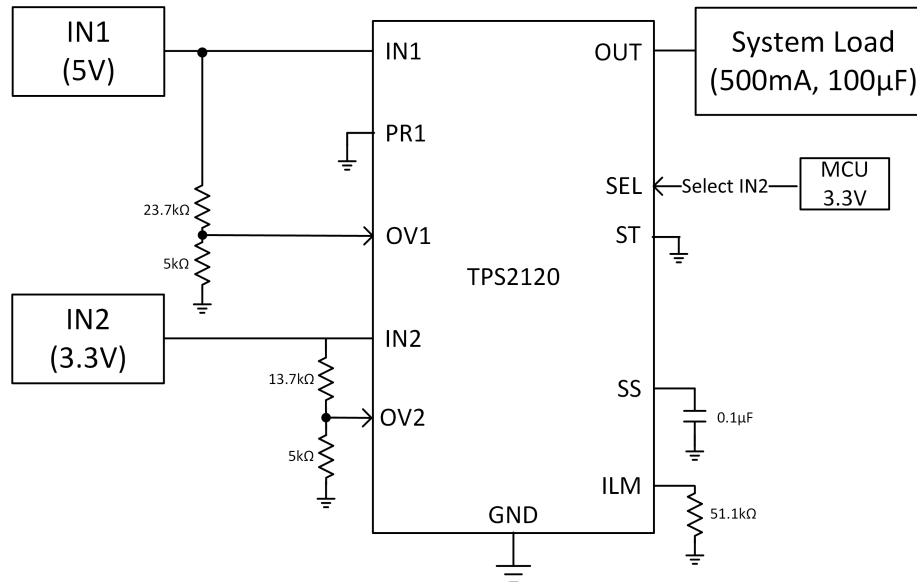
图 20. TPS2120 Manual Switchover
