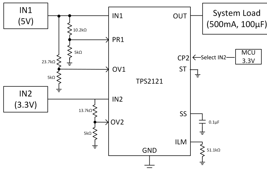
图 21. TPS2121 Manual Switchover
