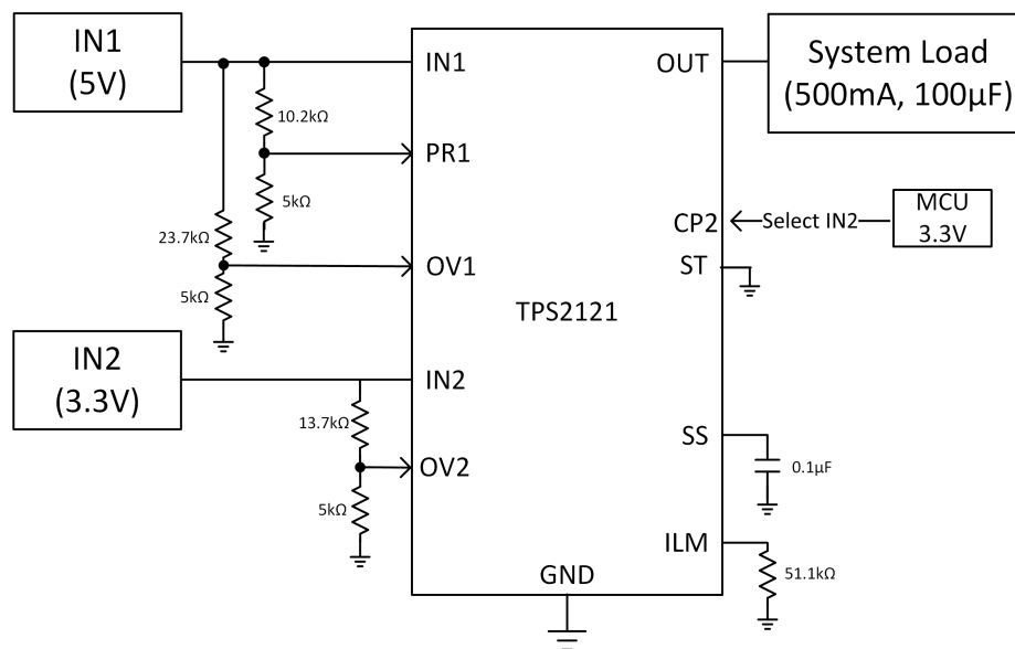
图 23. TPS2121 Manual Switchover
