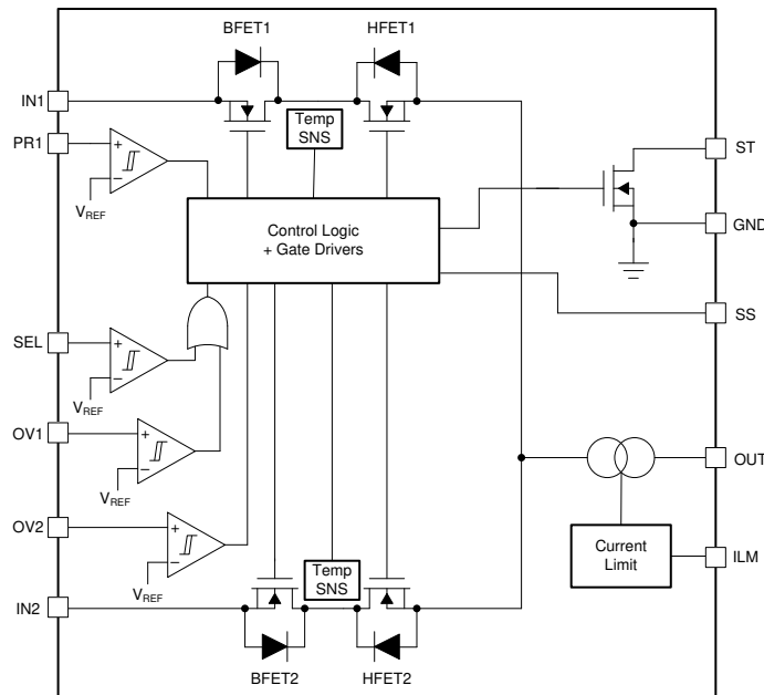
图 10. TPS2120 Functional Block Diagram
