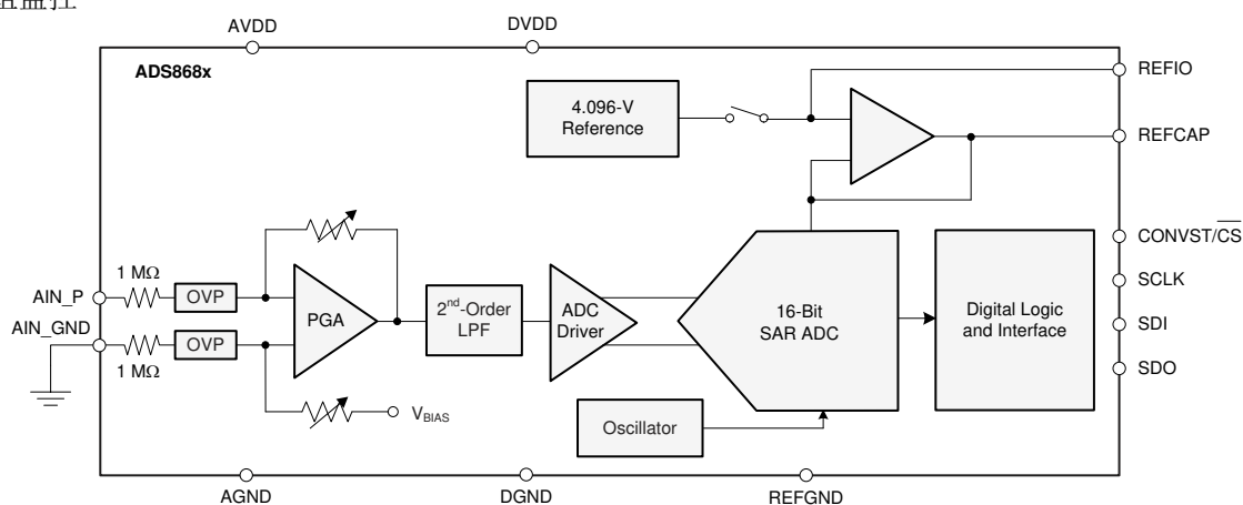
方框图
