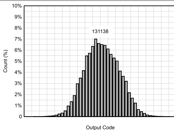
图 6-22. DC Histogram
