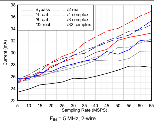
图 6-25. I_{IOVDD} Current vs Decimation
