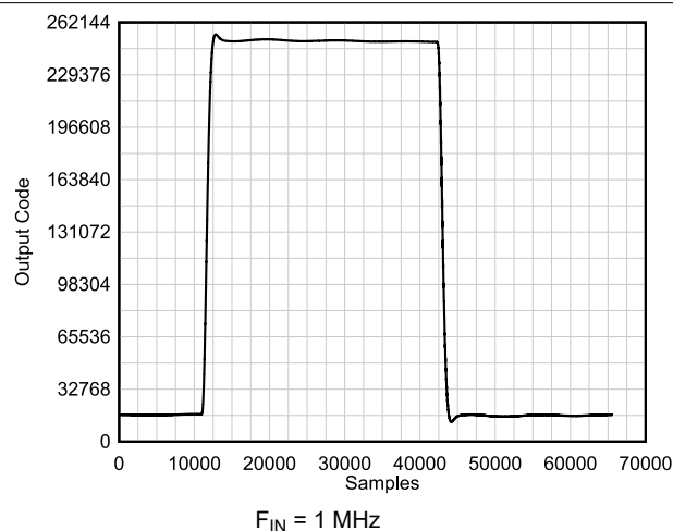
图 6-23. Pulse Response
