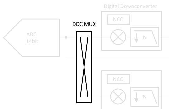
图 8-20. DDC MUX
