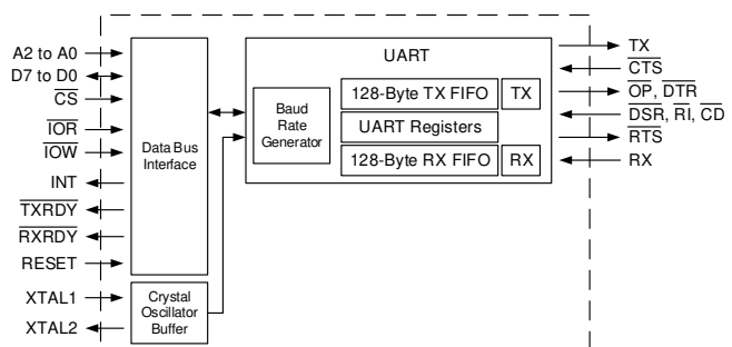
方框图
