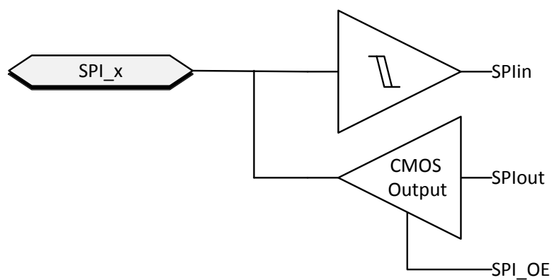
图 25. SPI buffer
