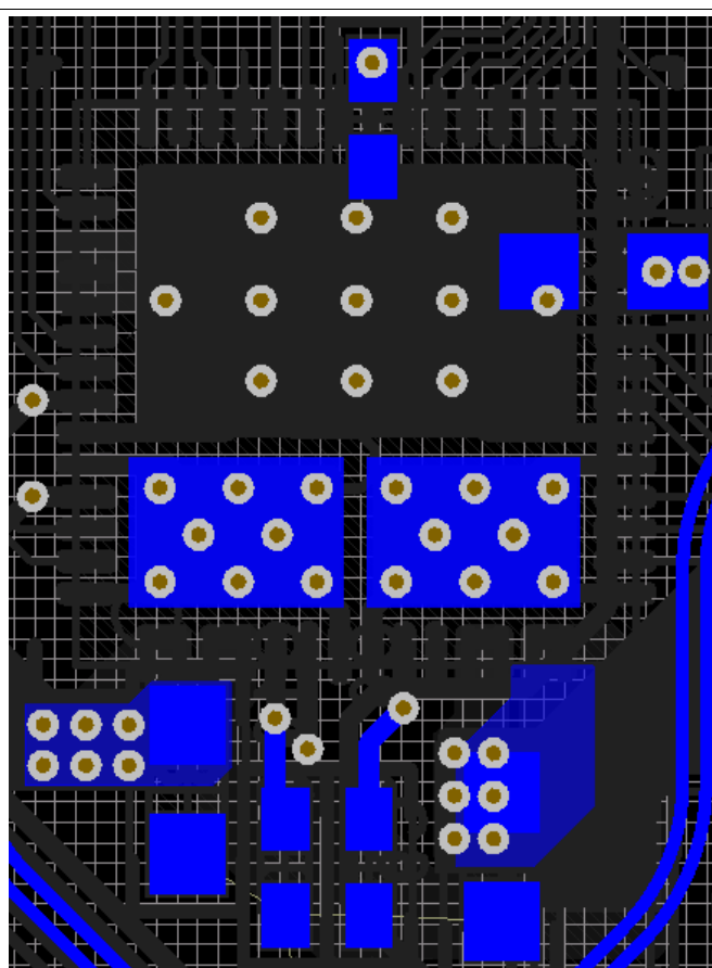
图 51. Bottom Polygon Pours
