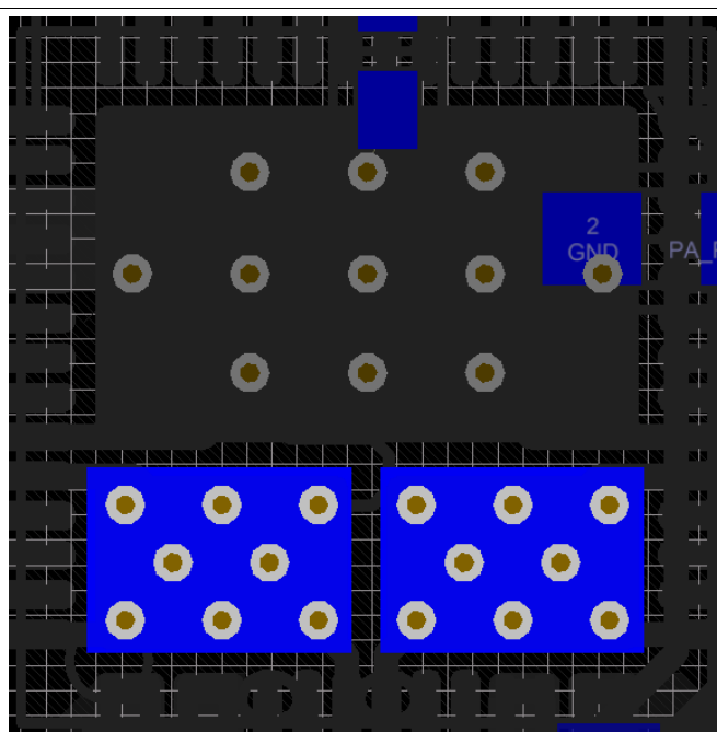
图 54. Bottom Layer FET Pads
