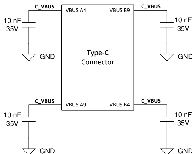
图 35. Type-C Connector VBUS Capacitors
