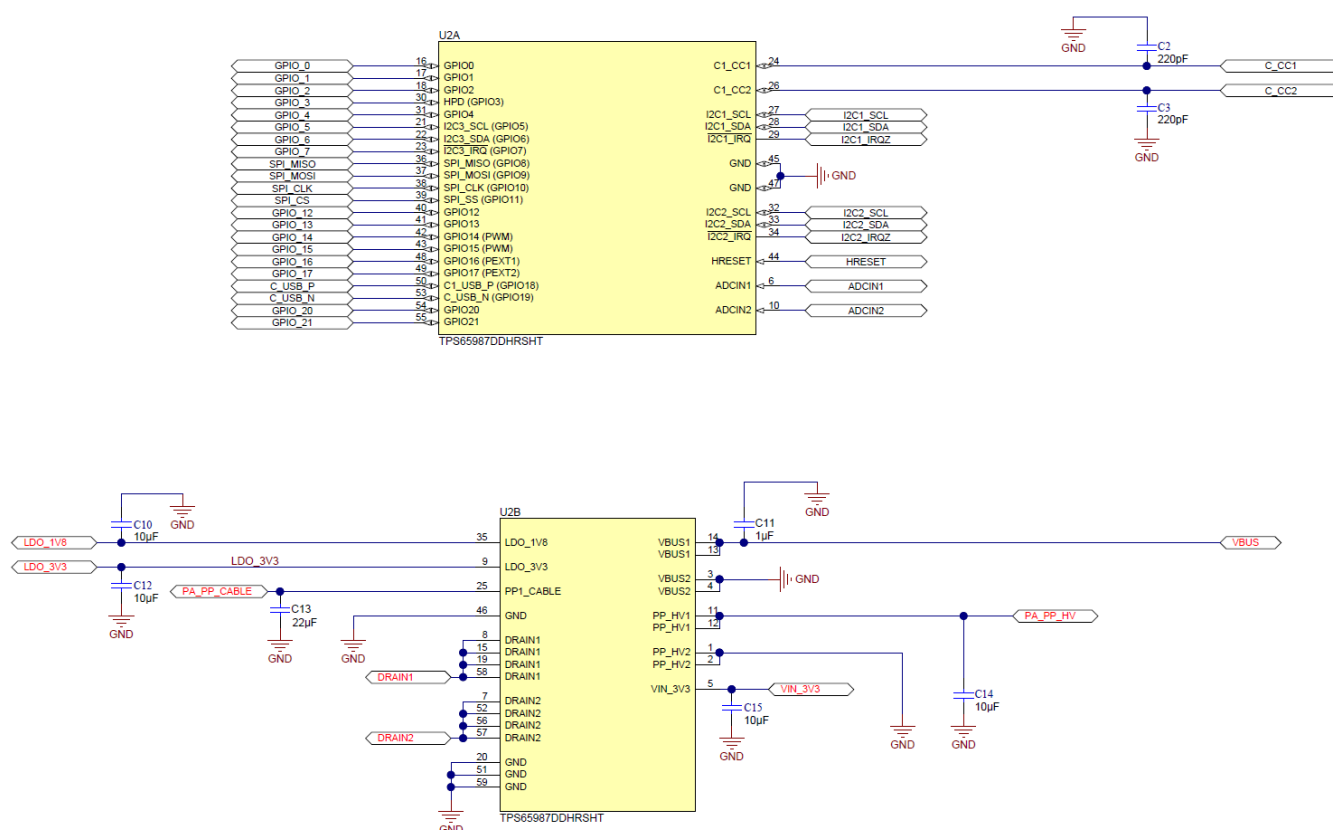
图 34. Example Schematic
