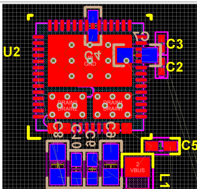
图 46. Bottom View Layout
