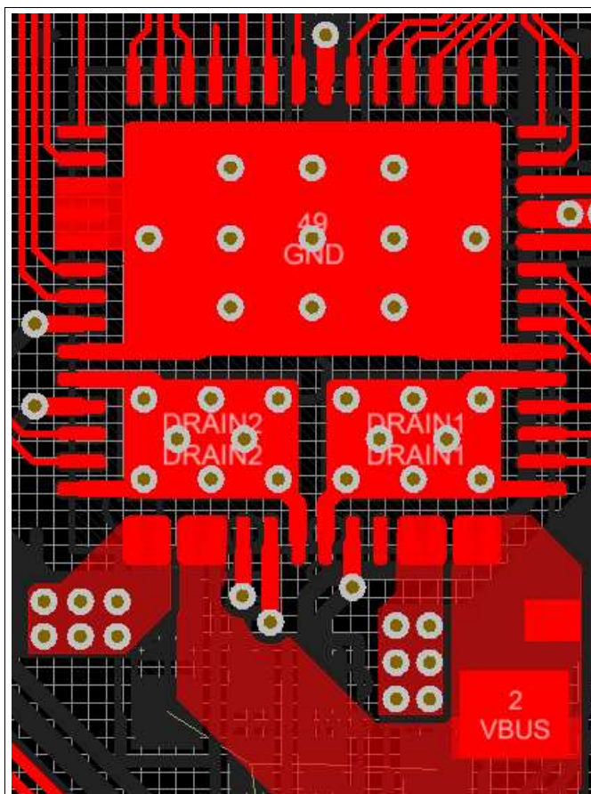
图 50. Top Polygon Pours
