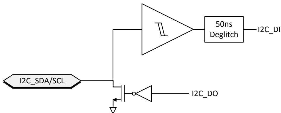
图 24. I 2 C Buffer
