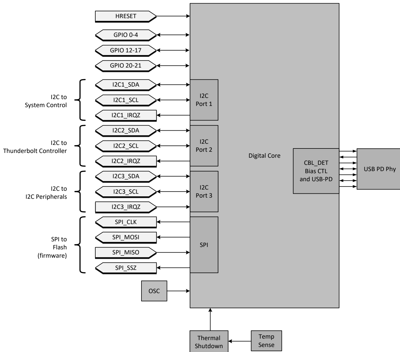
图 26. Digital Core Block Diagram
