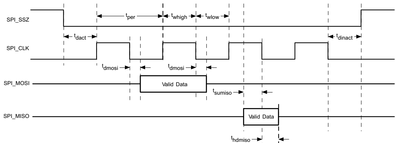
图 4. SPI Master Timing
