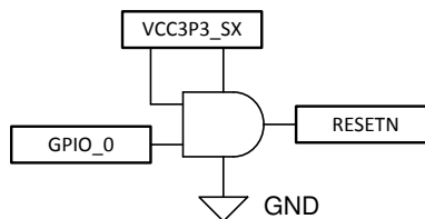
图 41. RESETN Circuit
