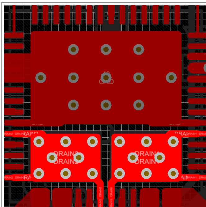
图 53. Top Layer FET Pads
