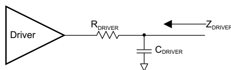
图 11. ZDRIVER Circuit
