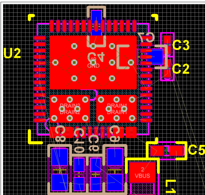
图 45. Top View Layout
