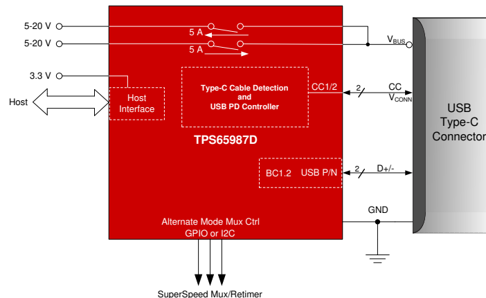
简化原理图
