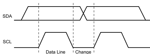
图 28. I 2 C Bit Transfer
