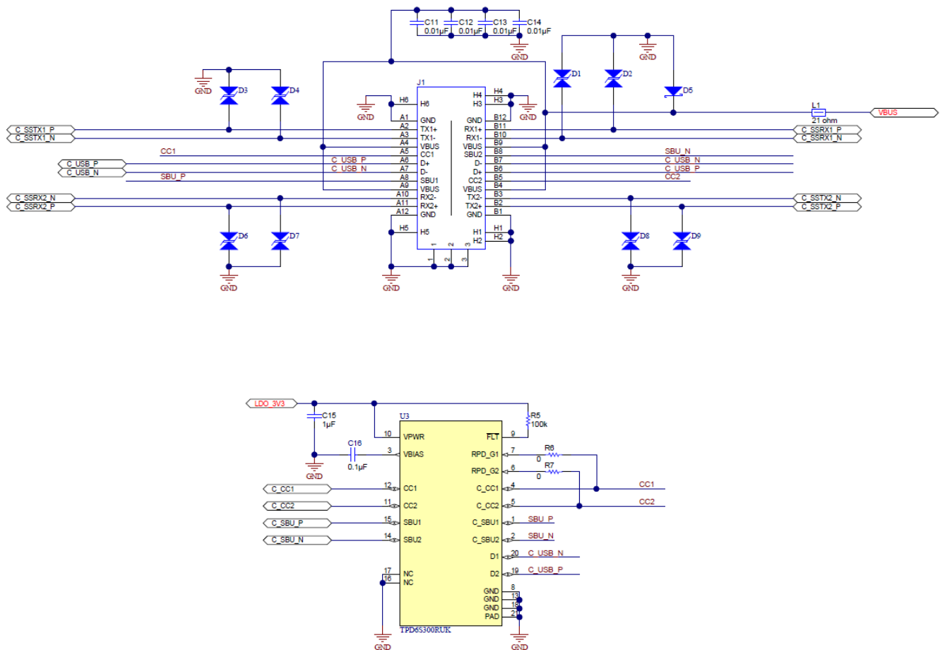
图 44. Example Schematic2
