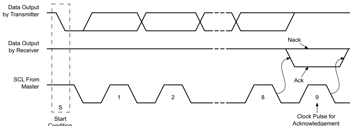
图 29. I 2 C Acknowledgment
