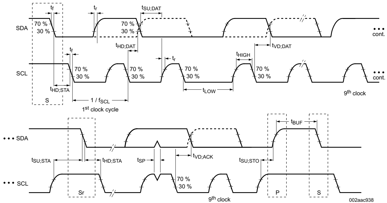
图 3. I²C Slave Interface Timing
