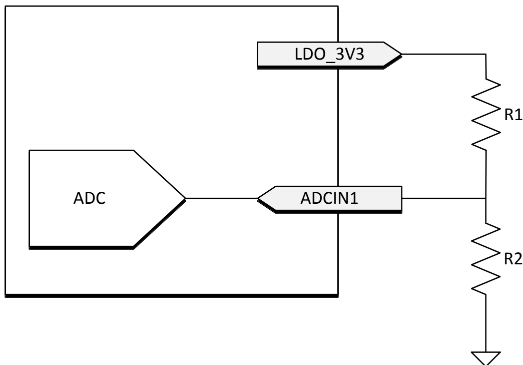
图 21. ADCIN1 Resistor Divider
