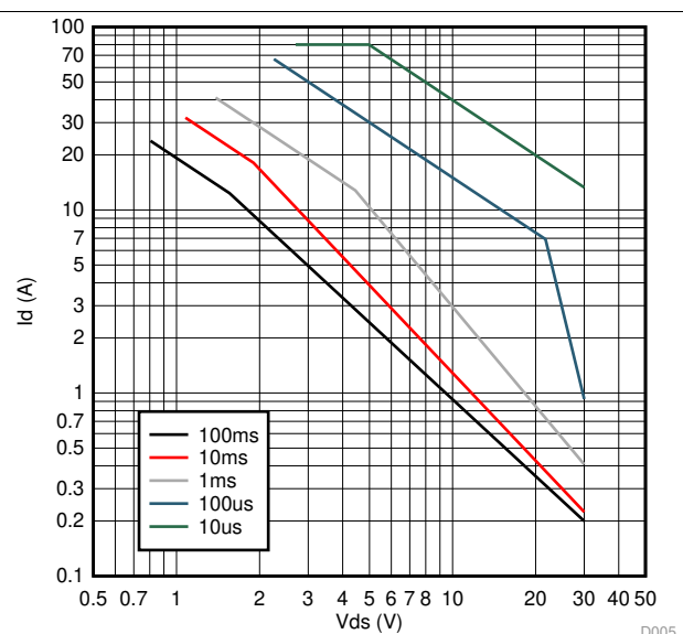
图 2. PPHVx SOA Curve
