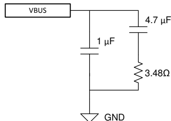
图 36. VBUS Snubber
