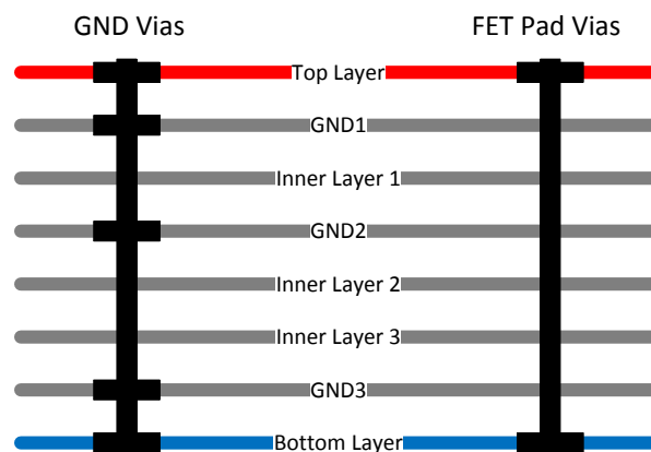
图 56. PCB Stack-Up
