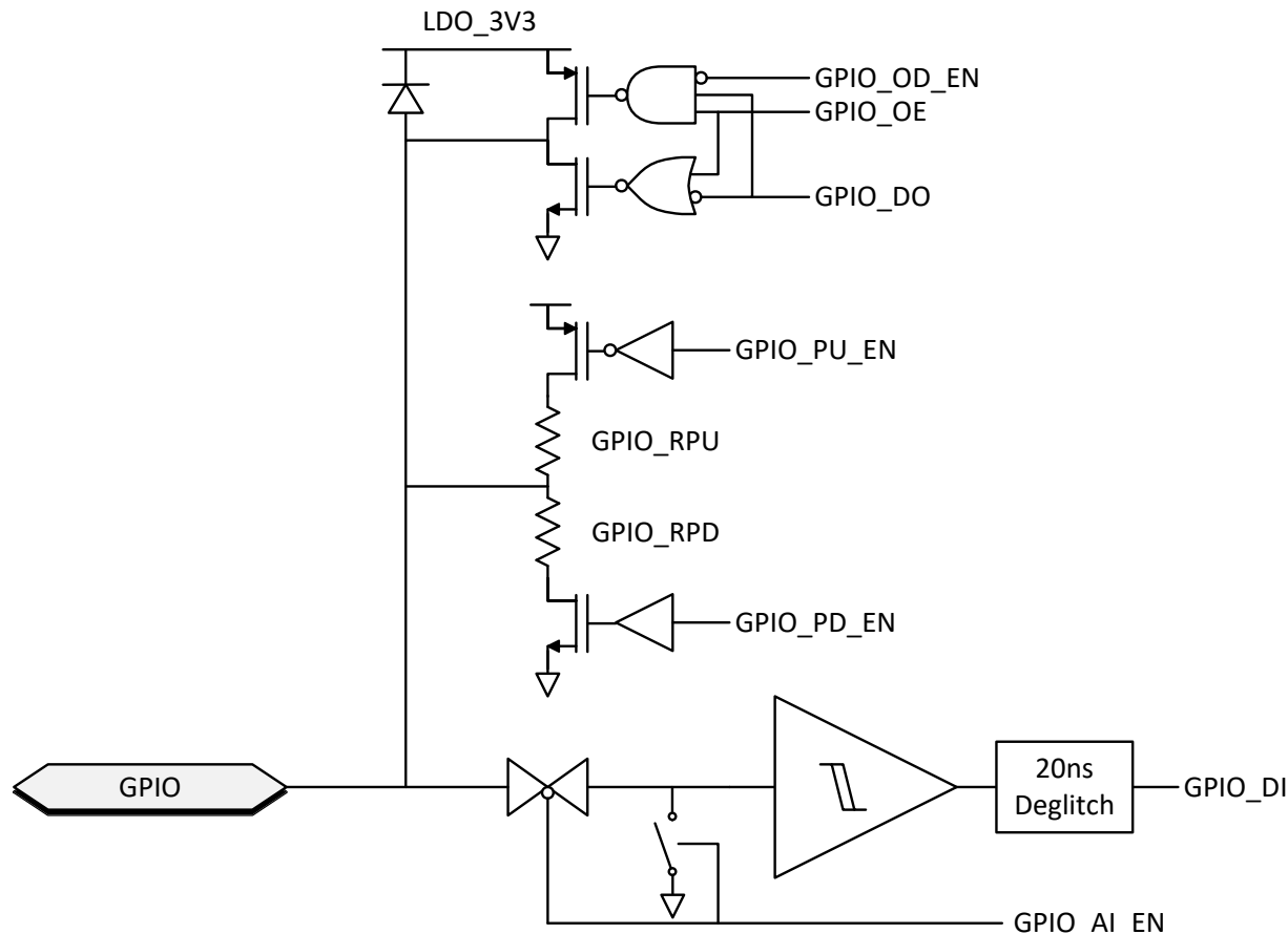
图 23. General GPIO Buffer
