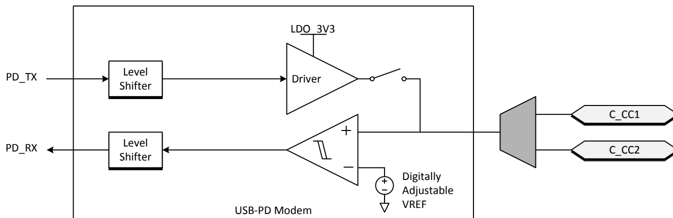
图 9. USB-PD BMC TX/Rx Block Diagram
