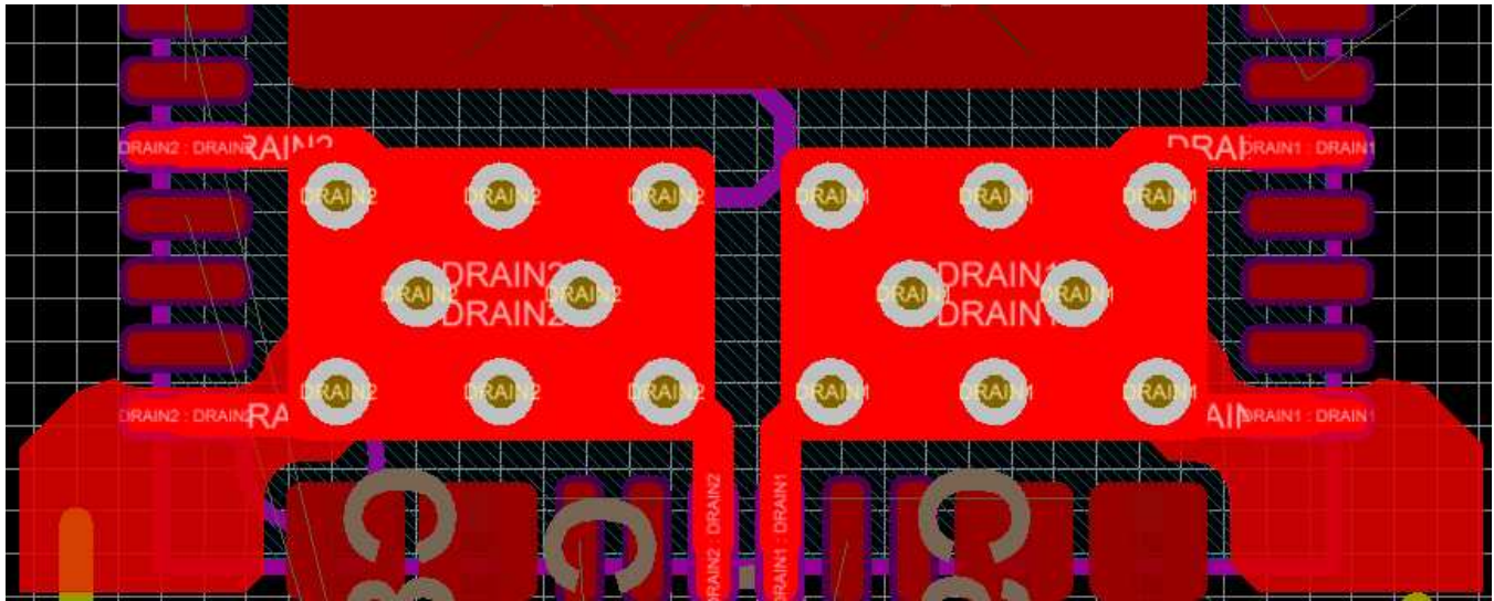
图 55. Copper Fins on Drain Pad
