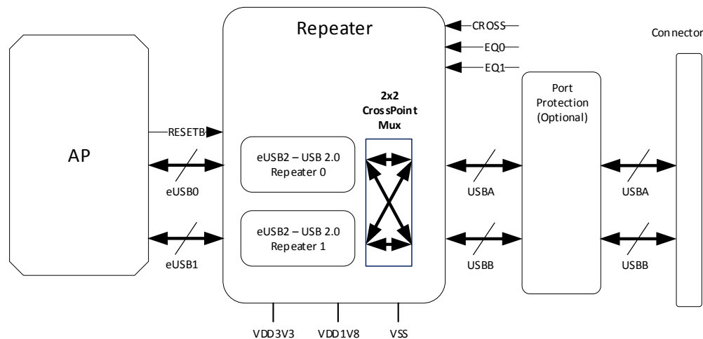
TUSB2E22
