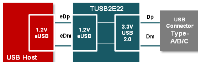
TUSB2E22
