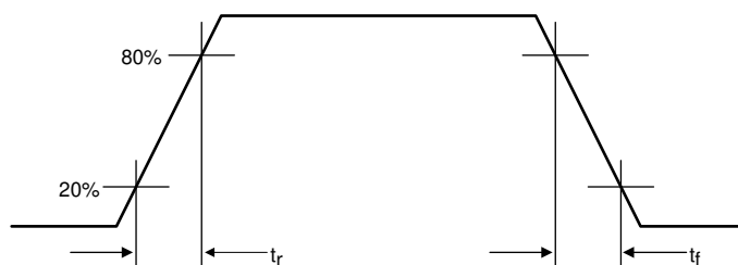
图 15. Output Rise and Fall Times
