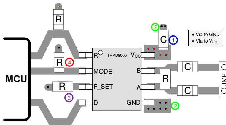
图 11-1. Layout Example (OOK)
