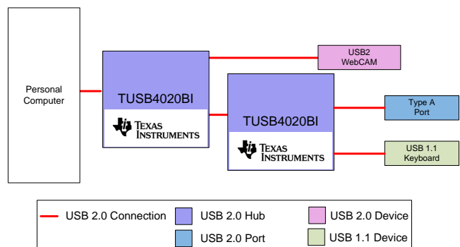
框图
