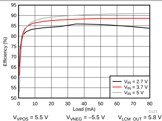
图 209. VPOS/VNEG Efficiency
