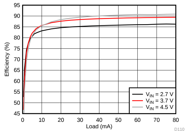
图 194. VPOS Efficiency
