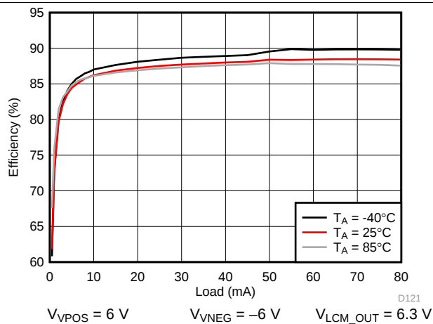
图 207. VPOS/VNEG Efficiency
