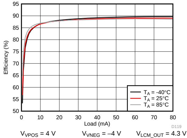
图 205. VPOS/VNEG Efficiency
