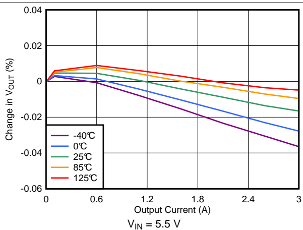
图 28. Load Regulation (5-V Output)
