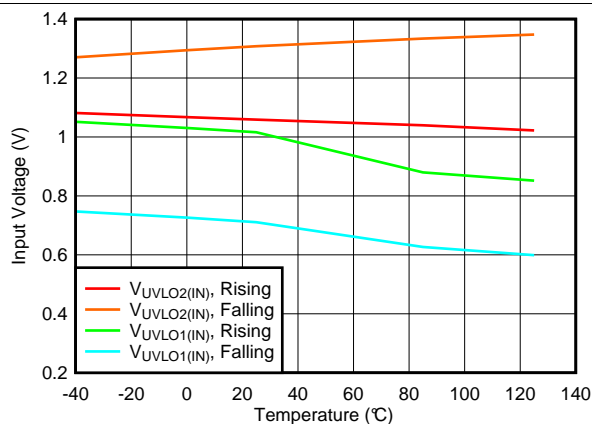
图 37. V_{IN} UVLO vs Temperature
