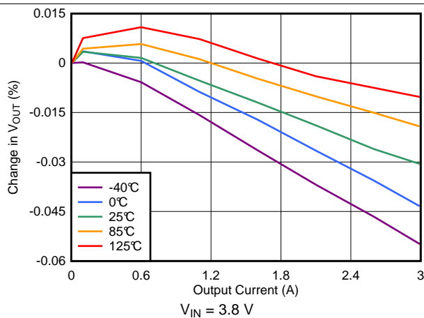
图 27. Load Regulation (3.3-V Output)
