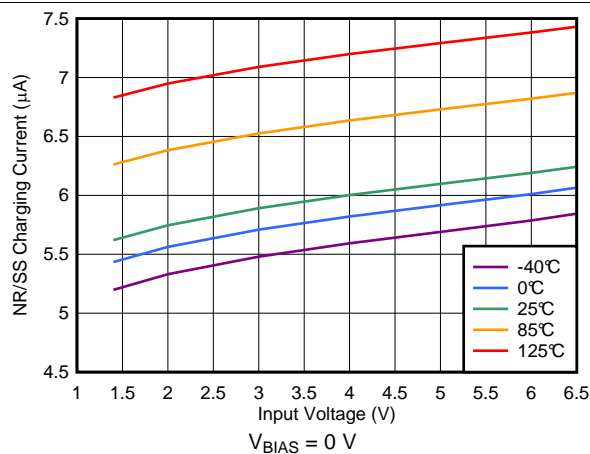
图 36. I_{NR/SS} Current vs Input Voltage
