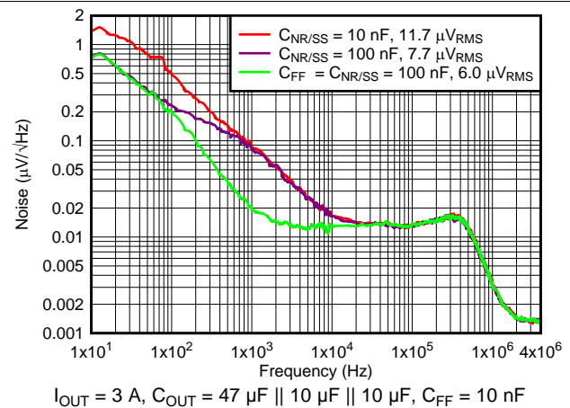
图 14. Output Noise at 5.0-V Output
