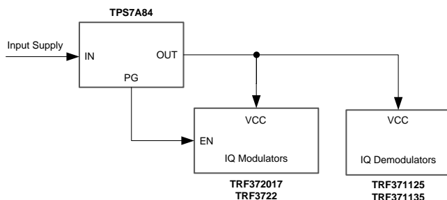
为 RF 组件供电
